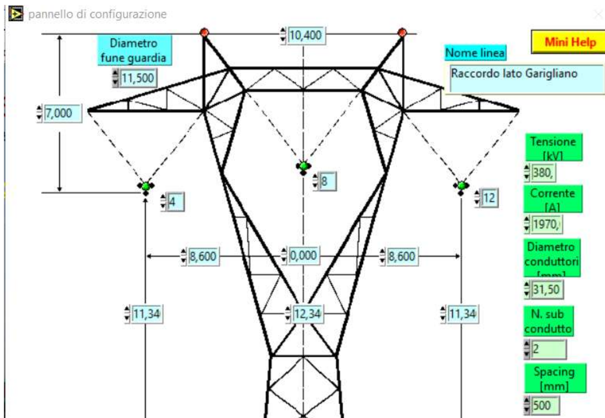
Fig.1 Configurazione di calcolo
