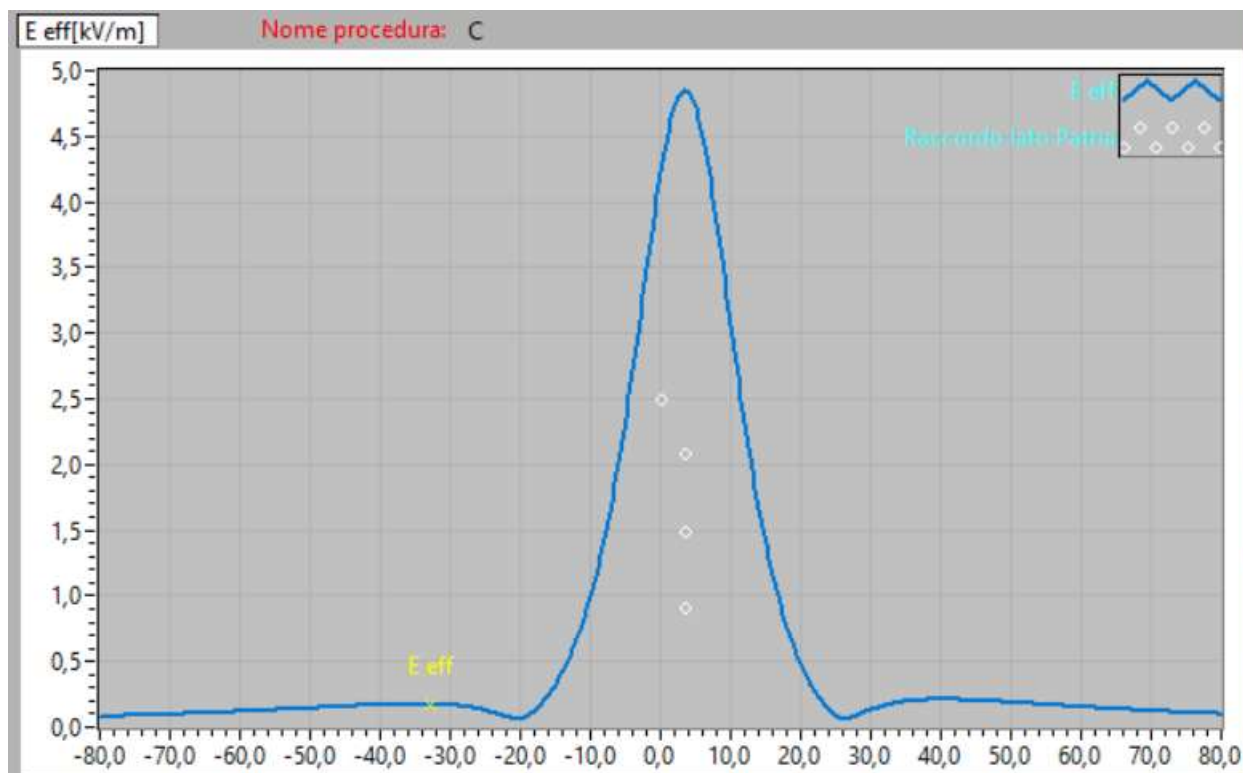
Fig.8 Grafico del campo elettrico
