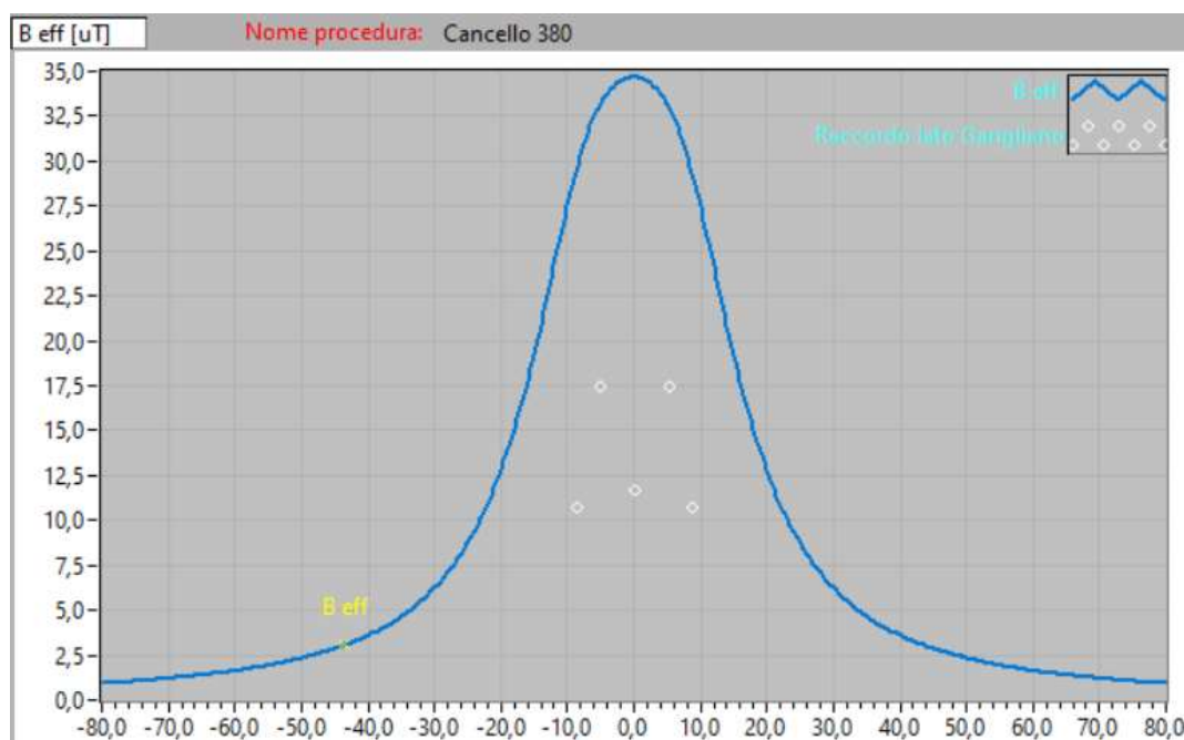
Fig.2 Grafico del campo magnetico ad 1 m dal suolo
