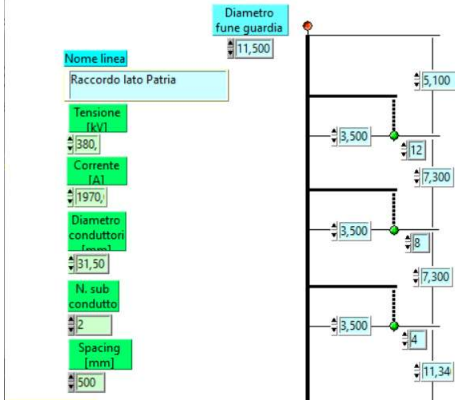
Fig.5 Configurazione di calcolo
