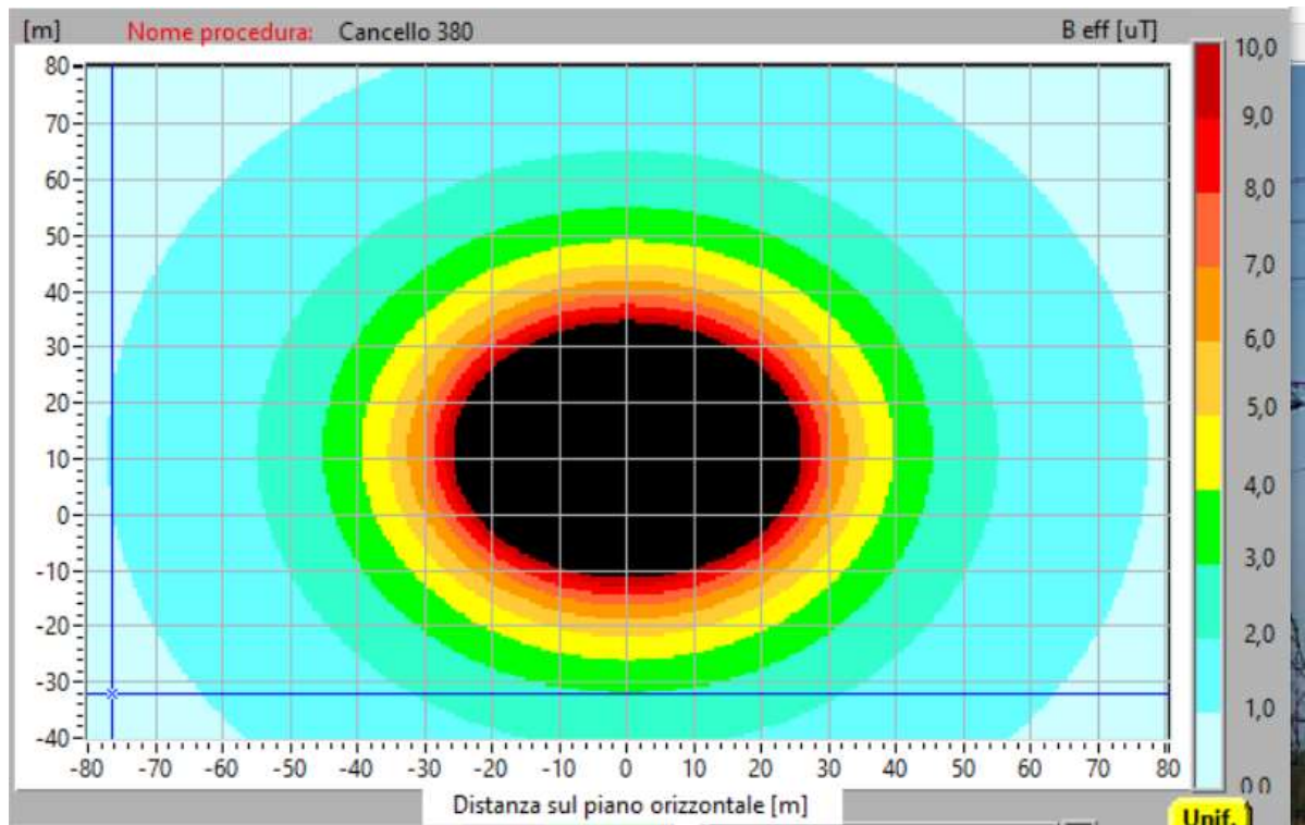
Fig.3 Grafico del campo magnetico a quota conduttori
