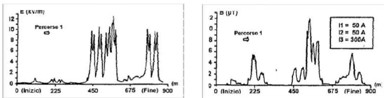
Figura 10 Risultati della misura dei campi elettrici e magnetici effettuate lungo le vie interne della sezione a 380 kV della stazione riportata in fig. 9
