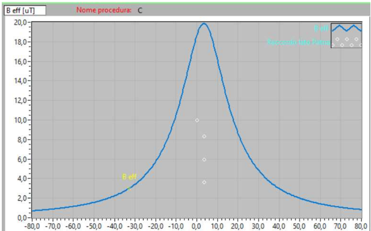
Fig.6 Grafico del campo magnetico ad 1 m dal suolo
