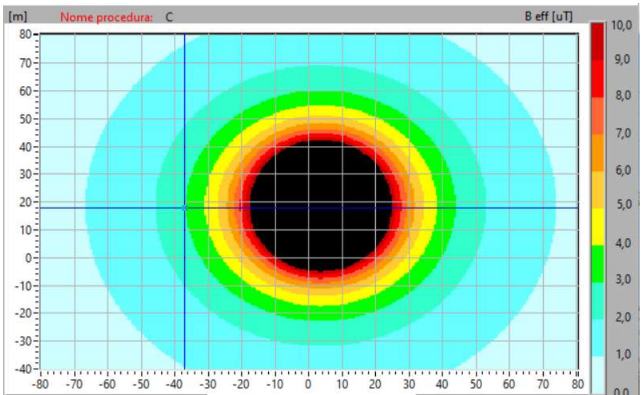
Fig.7 Grafico del campo magnetico a quota conduttori
