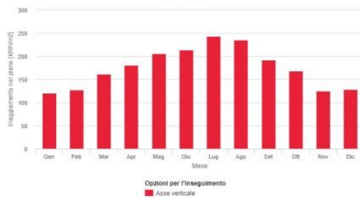
Figura 15: irraggiamento /energia media mensile
