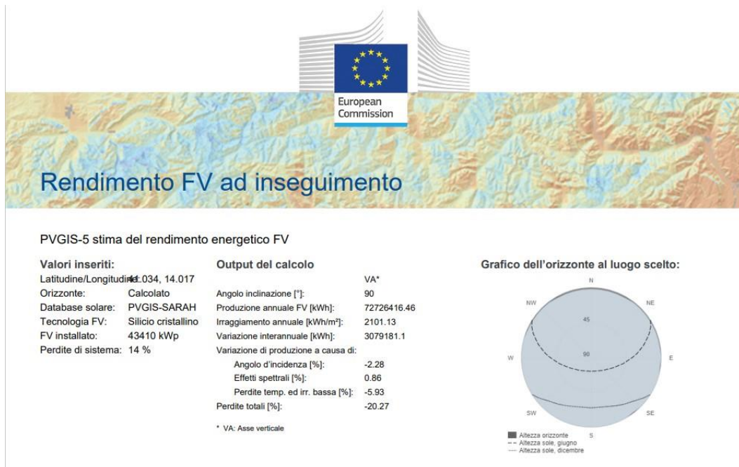
Figura 16: rendimento impianto
