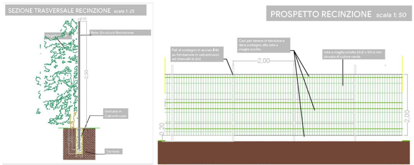
Figura 12: particolare recinzione
