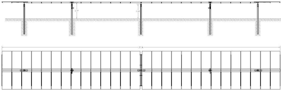
Figura 5: Struttura di Supporto – inseguitori mono assiali per i moduli fotovoltaici da 28 e da 56 moduli fv.
