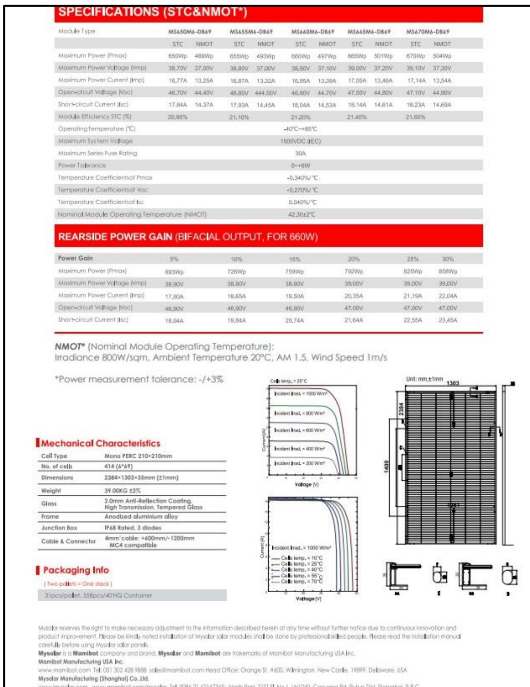
Figura 4: Scheda elettrica modulo fotovoltaico
