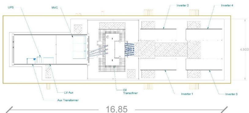
Figura 7: Power station con massimo 4 inverters centralizzati
