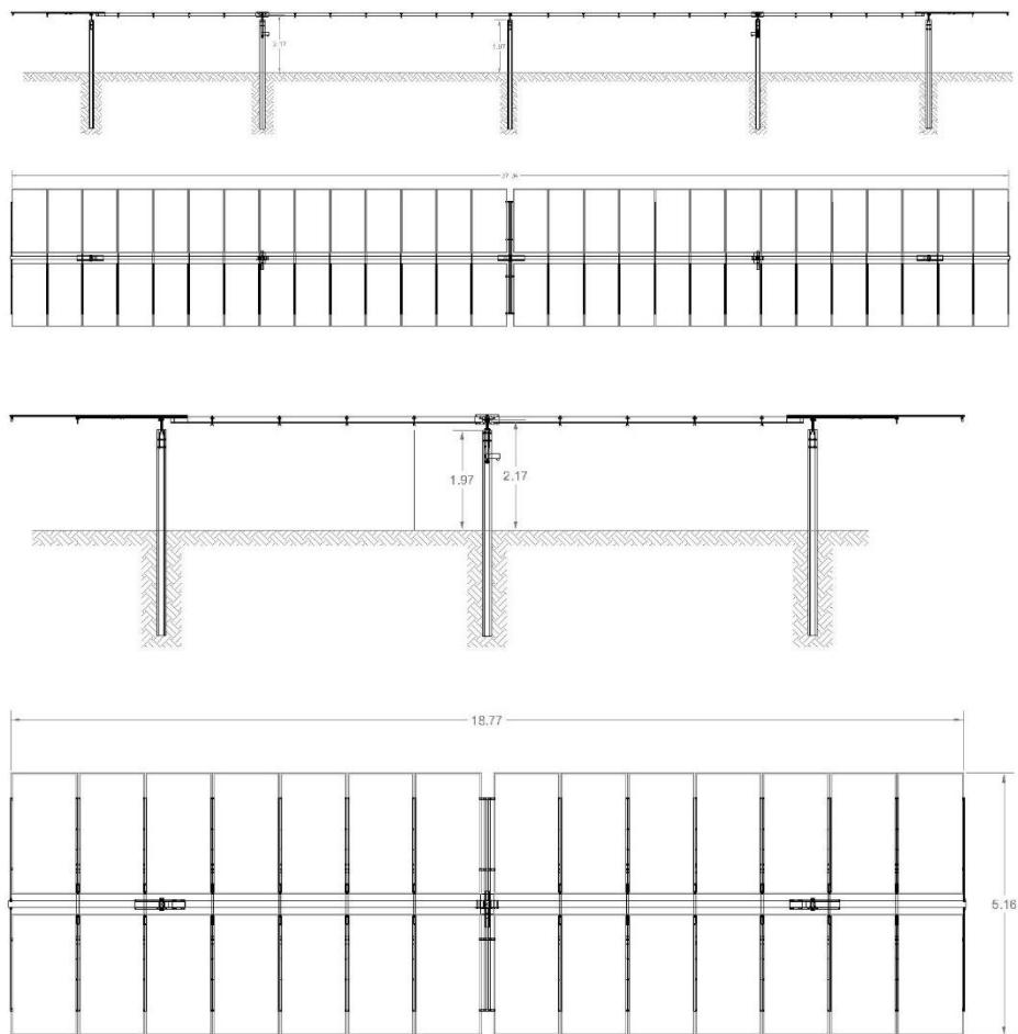
Figura 9: Strutture di supporto (trackers)
