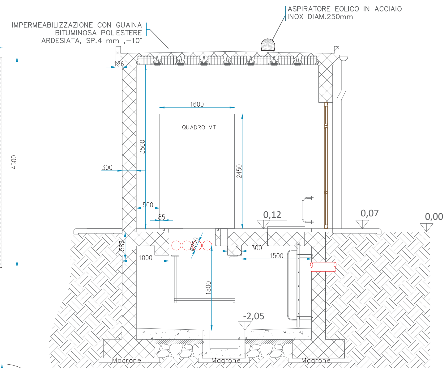
SEZIONE A-A
