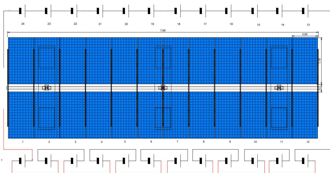
Fig. 04 - stringa in doppia fila 2x12 portrait
