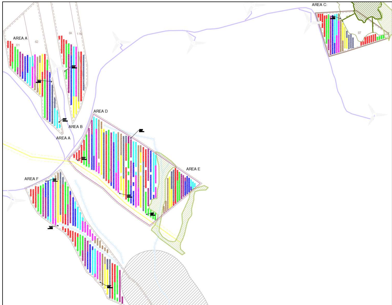
Fig. 03 - Layout impianto su rilievo topografico
