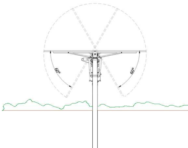
Fig 05 - esempio di inseguitore "Tracker"
