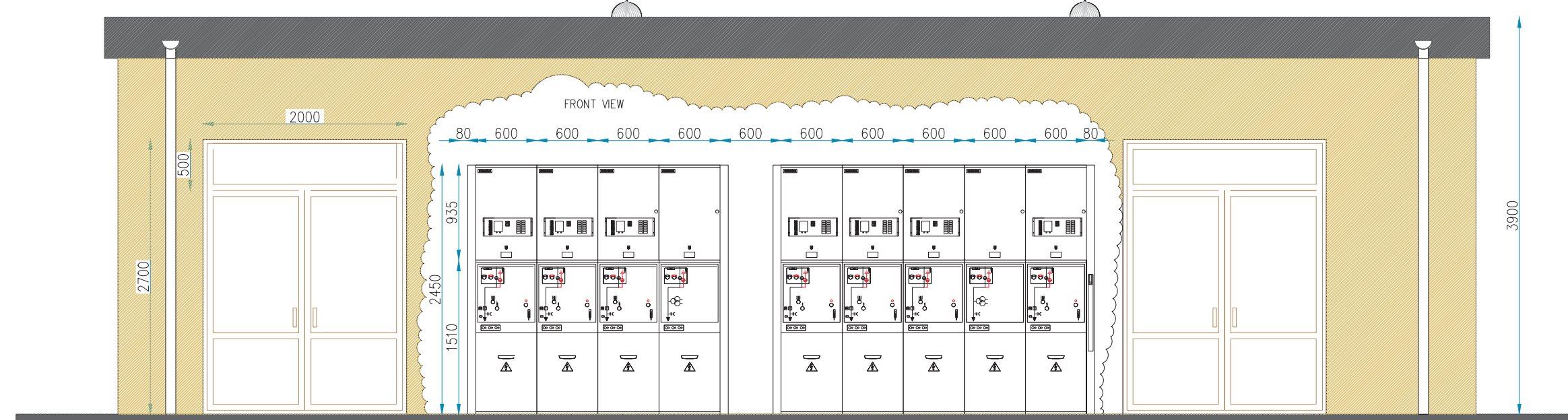
PROSPETTO ANTERIORE
