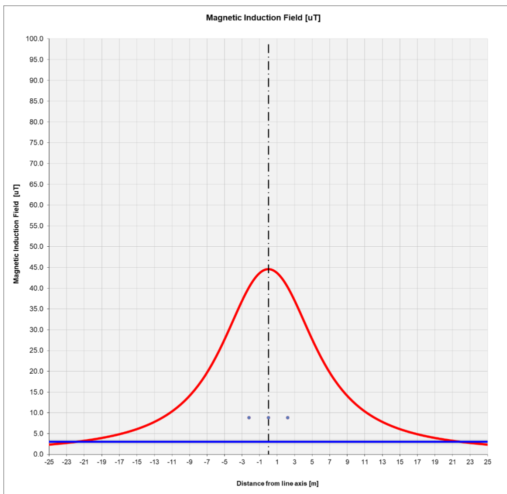
Figura 7: Andamento del campo di induzione magnetica per I = 2000 \text{ A}
