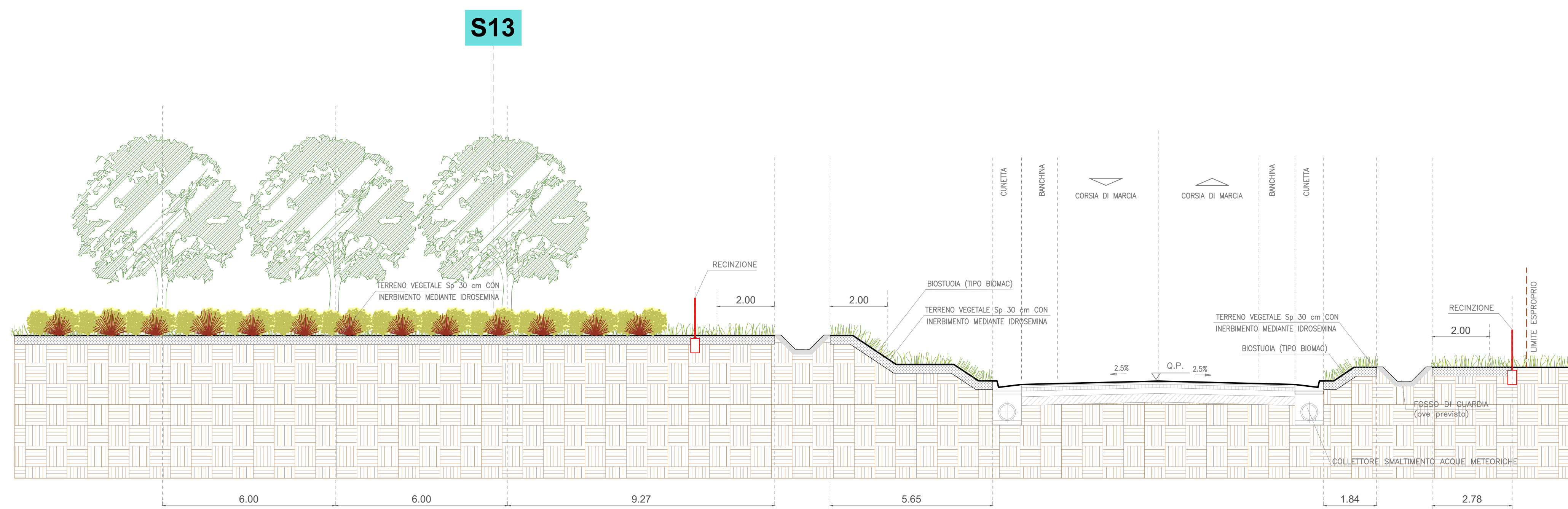
SEZIONE D-D'
