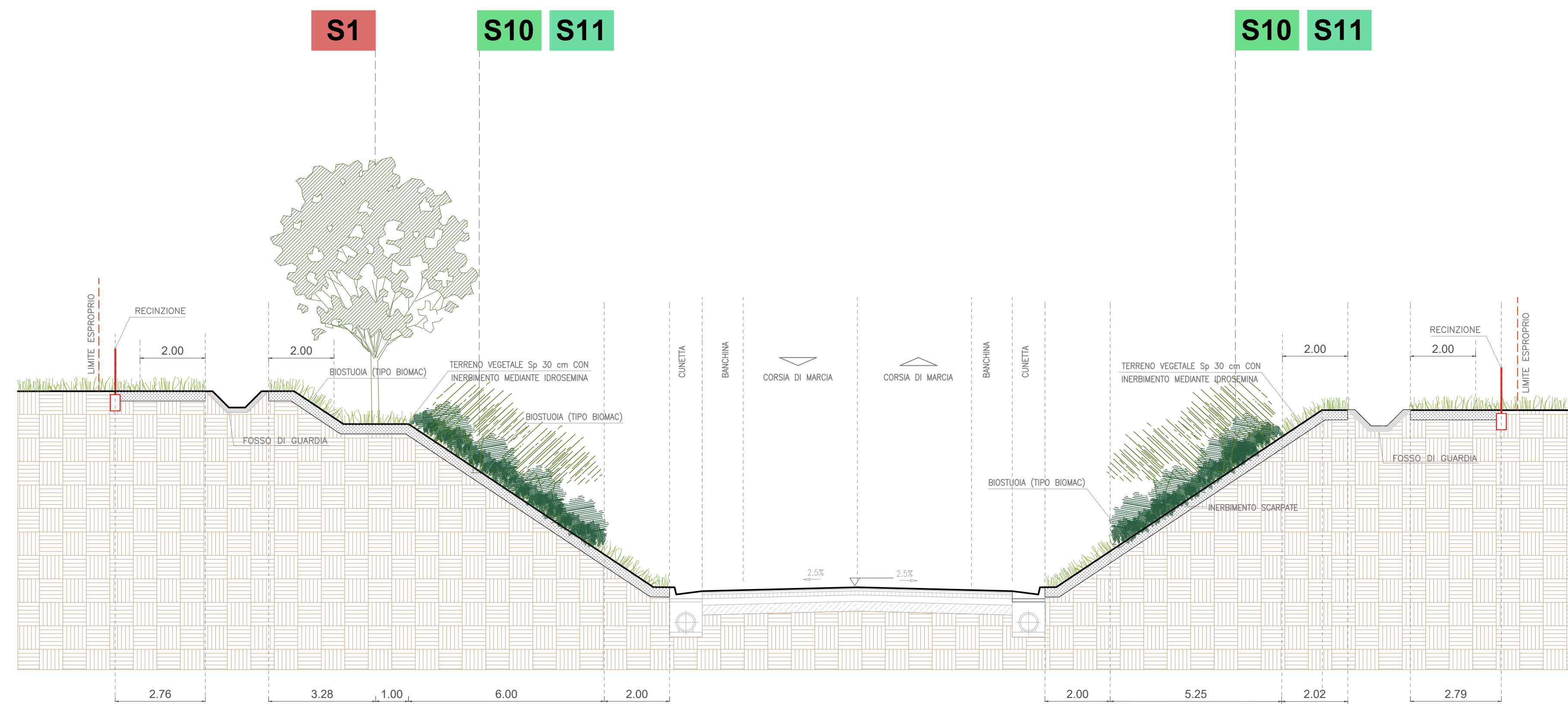
SEZIONE A-A'
