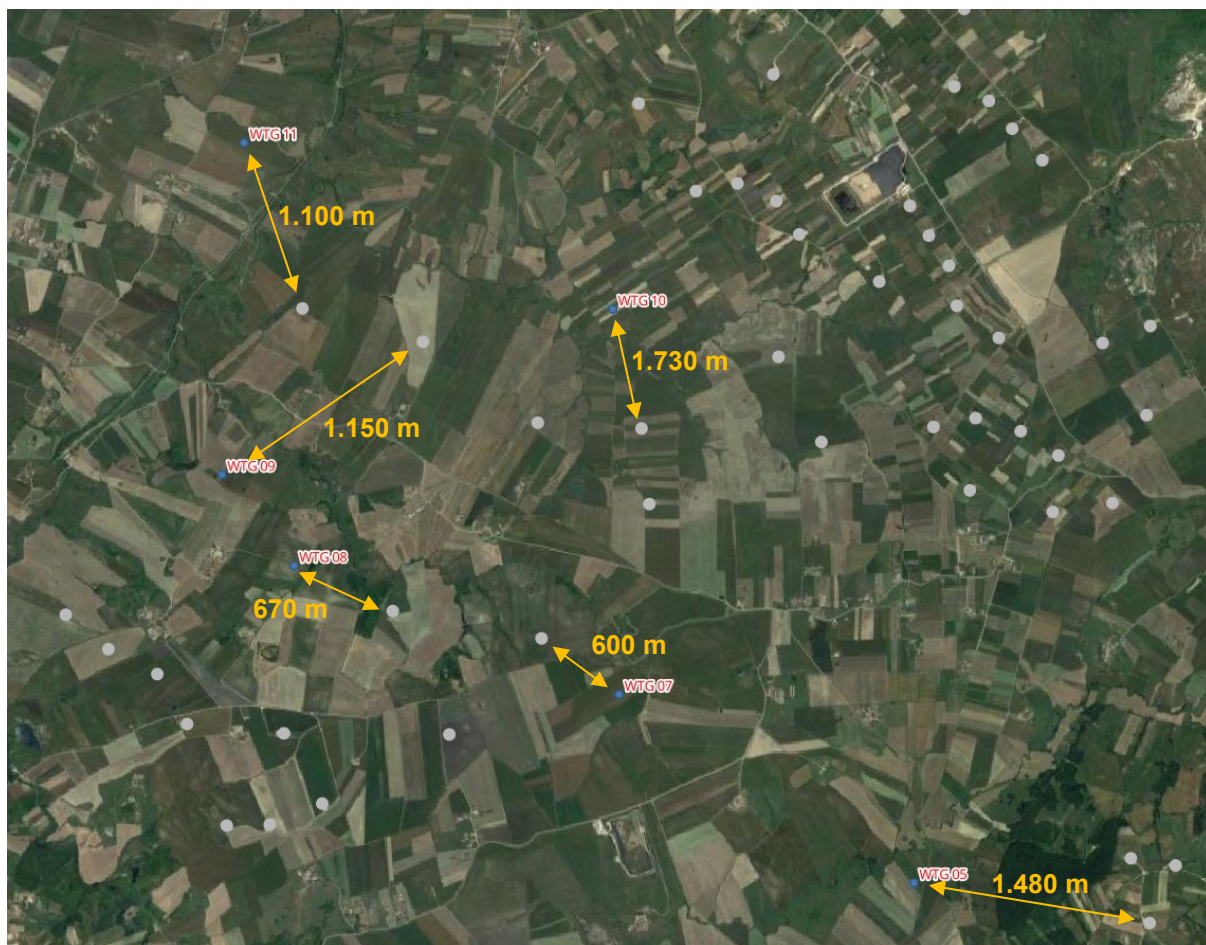
Figura 7 – Distanza tra gli aerogeneratori WTG 05-07-08-09-10-11 e altre ditte (in grigio quelli esistenti e in arancio quelli approvati)
