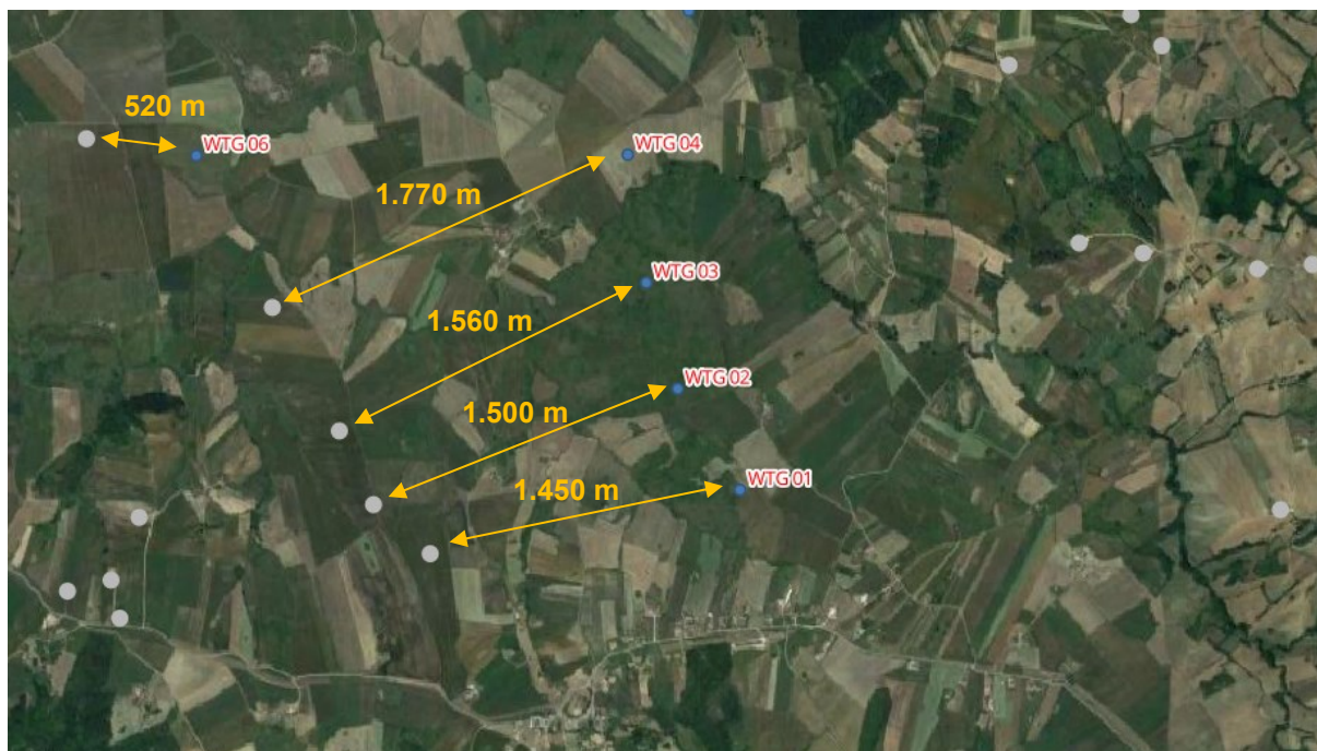
Figura 8 – Distanza tra gli aerogeneratori WTG 01-02-03-04-06 e altre ditte (in grigio quelli esistenti e in arancio quelli approvati)
