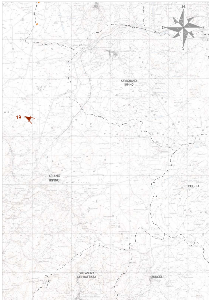
Punto di osservazione n° 19 - Vista Sud-Est Regio tratturo Pescasseroli Candela [2] _ Comune di Ariano Irpino Stato di fatto
