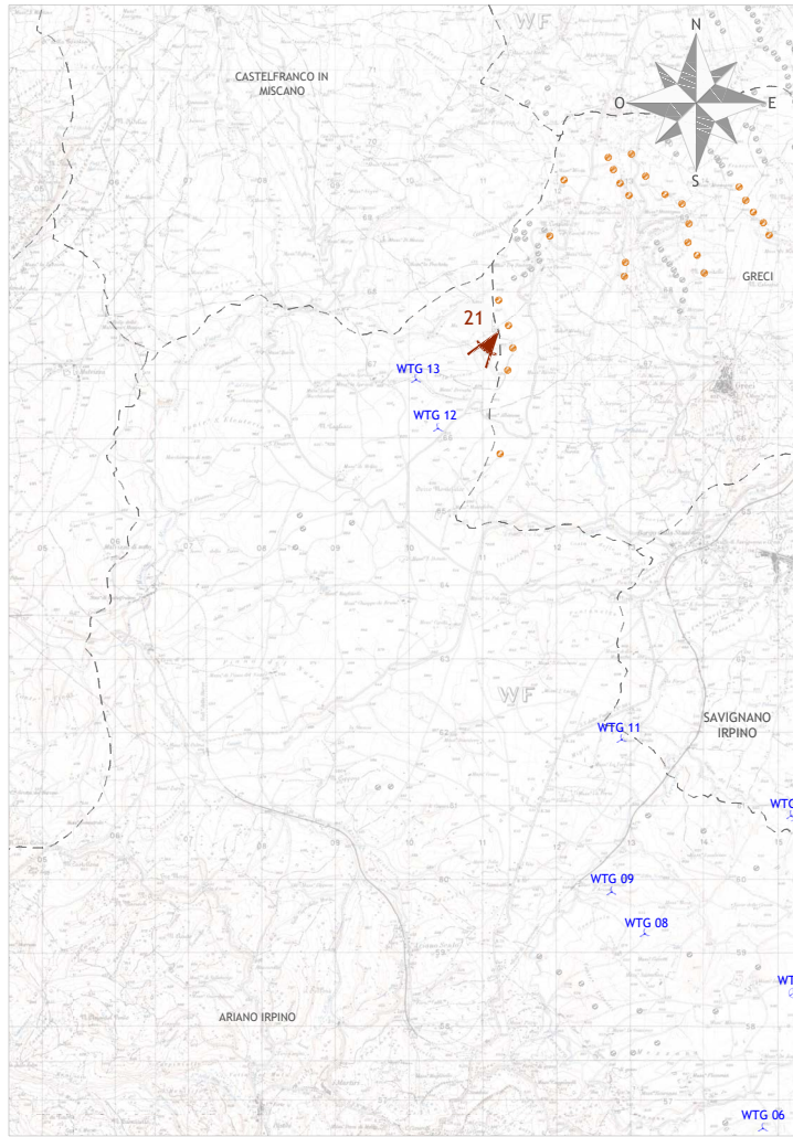
Punto di osservazione n°21 Tratturello Foggia Camporeale [2] _ Comune di Ariano Irpino Simulazione con impianto eolico
