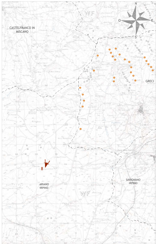
Punto di osservazione n°8 - Vista Nord-Est Masseria Chiuppo de Bruno con annessa cappella _ Comune di Ariano Irpino Stato di fatto
