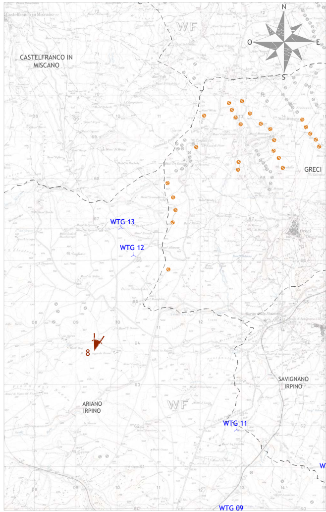
Punto di osservazione n°8 - Vista Nord-Est Masseria Chiuppo de Bruno con annessa cappella _ Comune di Ariano Irpino Simulazione con impianto eolico
