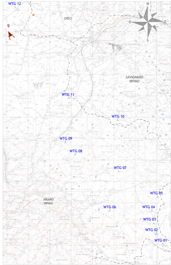
Punto di osservazione n° 9 - Vista Sud-Est Masseria Montefalco - Comune di Ariano Irpino Simulazione con impianto eolico
