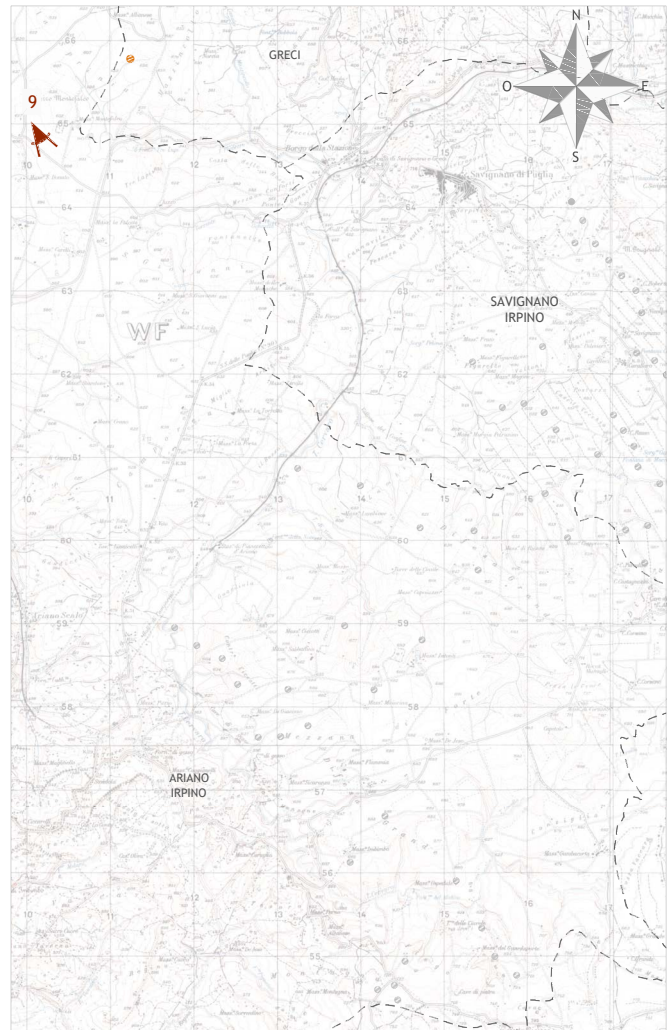
Punto di osservazione n° 9 - Vista Sud-Est Masseria Montefalco - Comune di Ariano Irpino Stato di fatto
