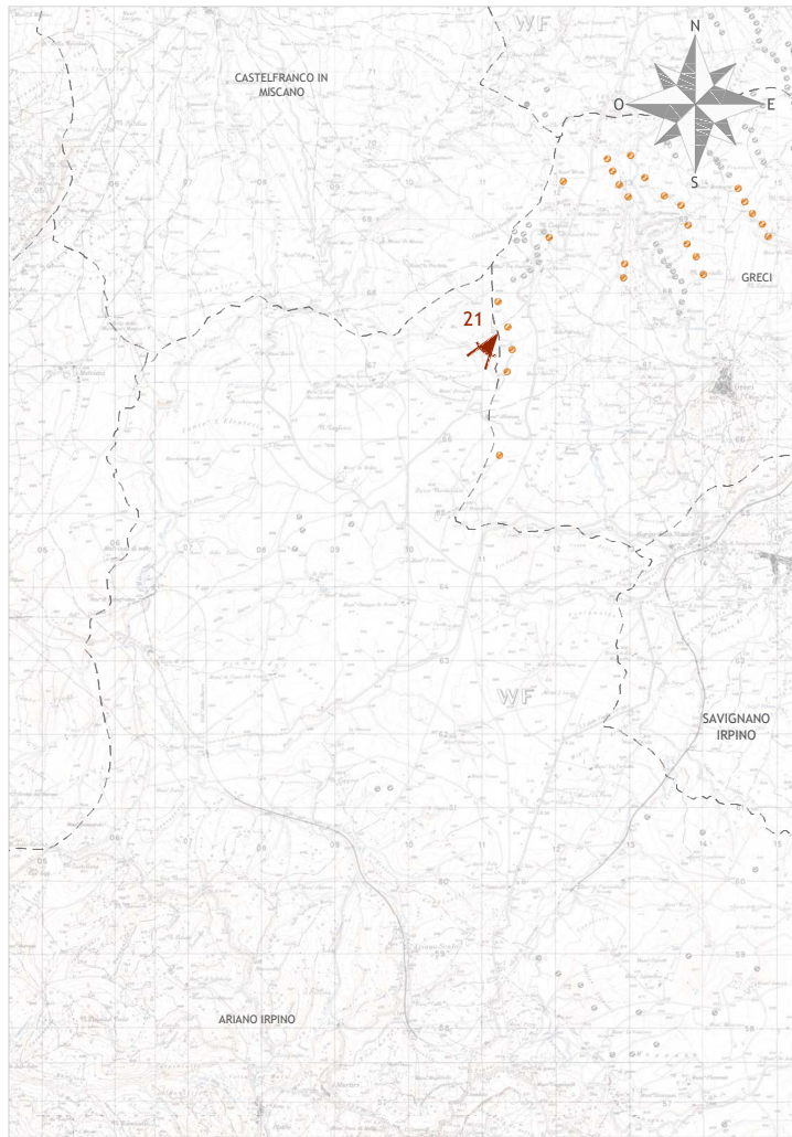
Punto di osservazione n°21 Tratturello Foggia Camporeale [2] _ Comune di Ariano Irpino Stato di fatto
