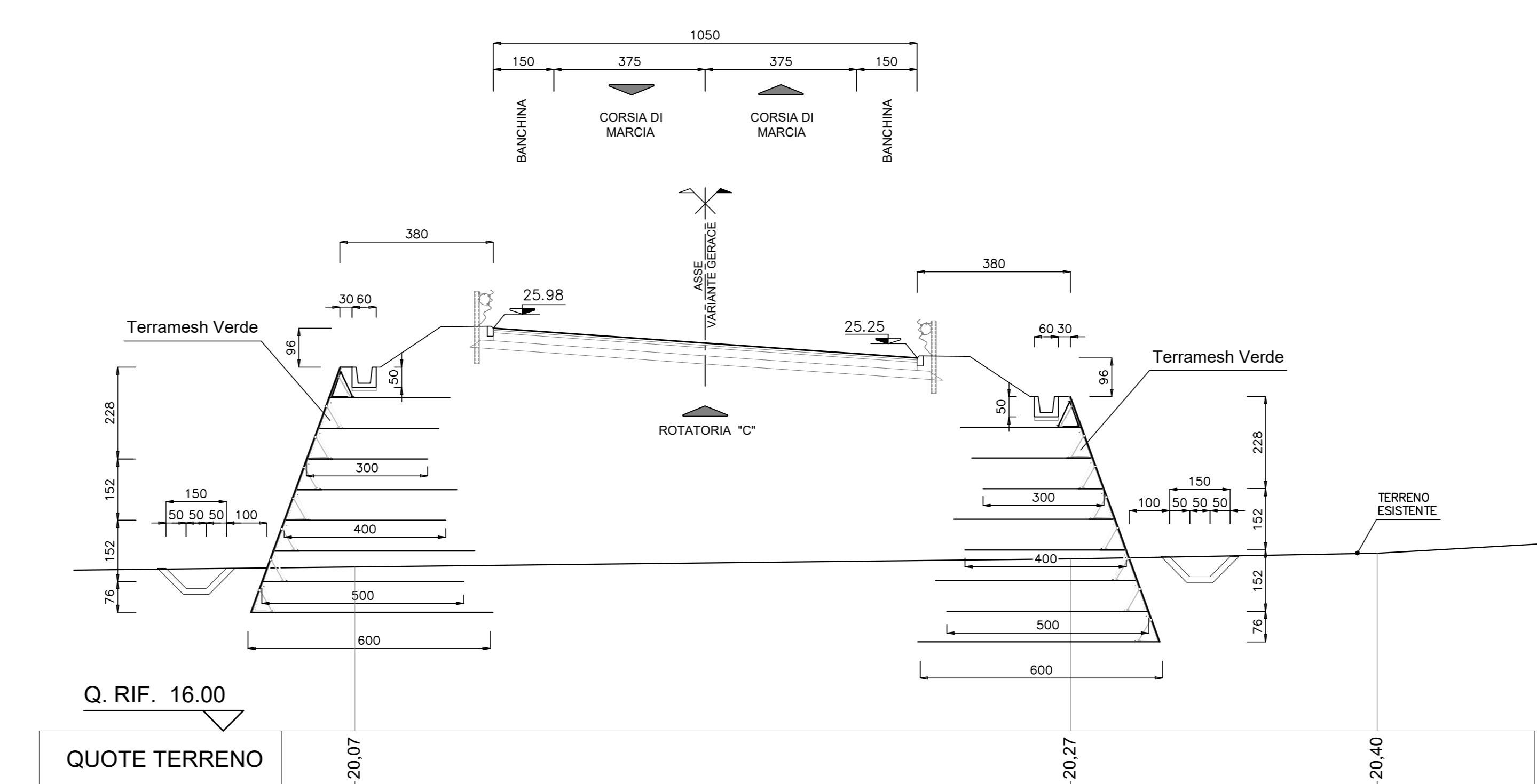
SEZIONE A PRG. 480.00
