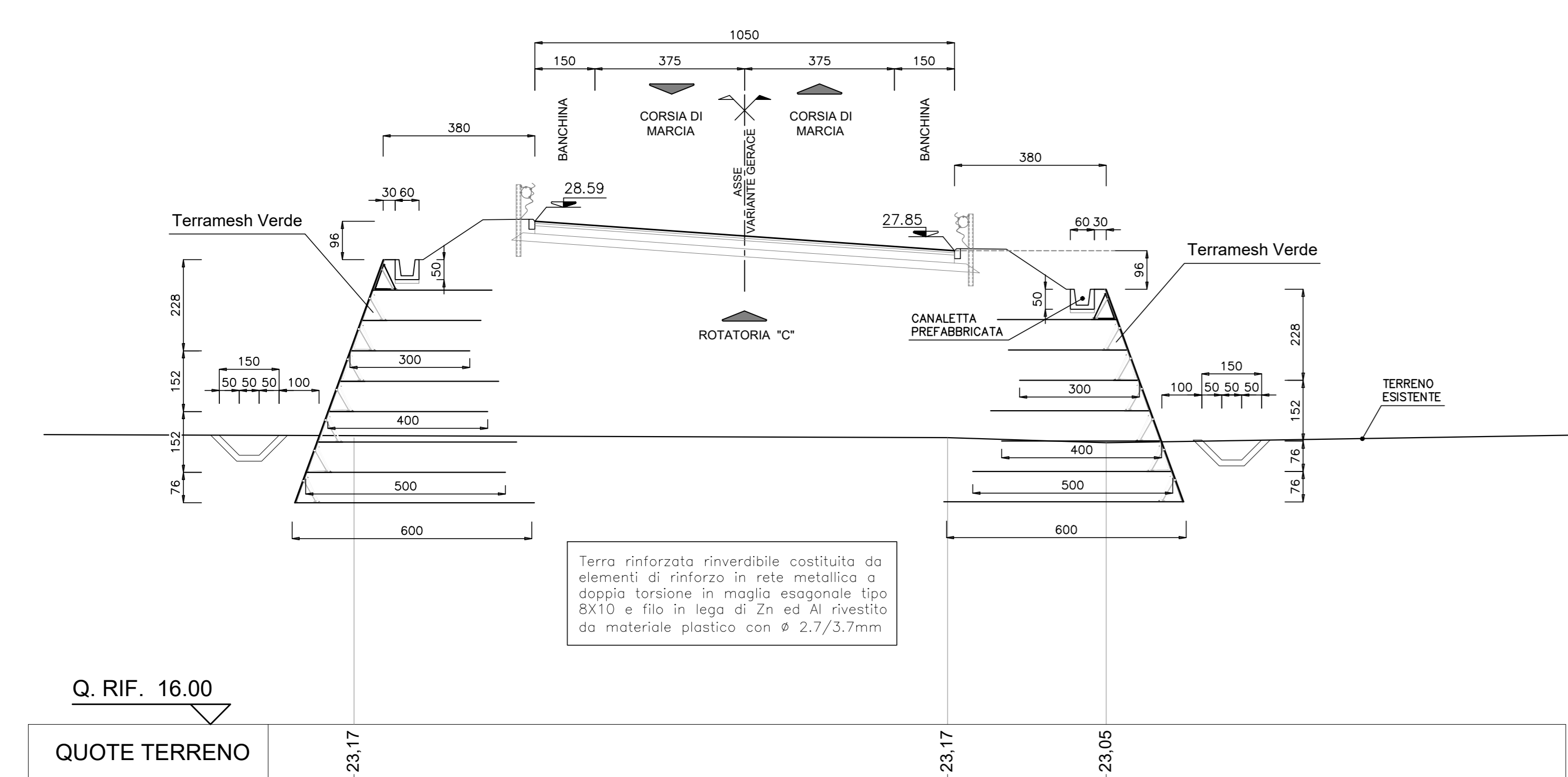
SEZIONE A PRG. 440.00
