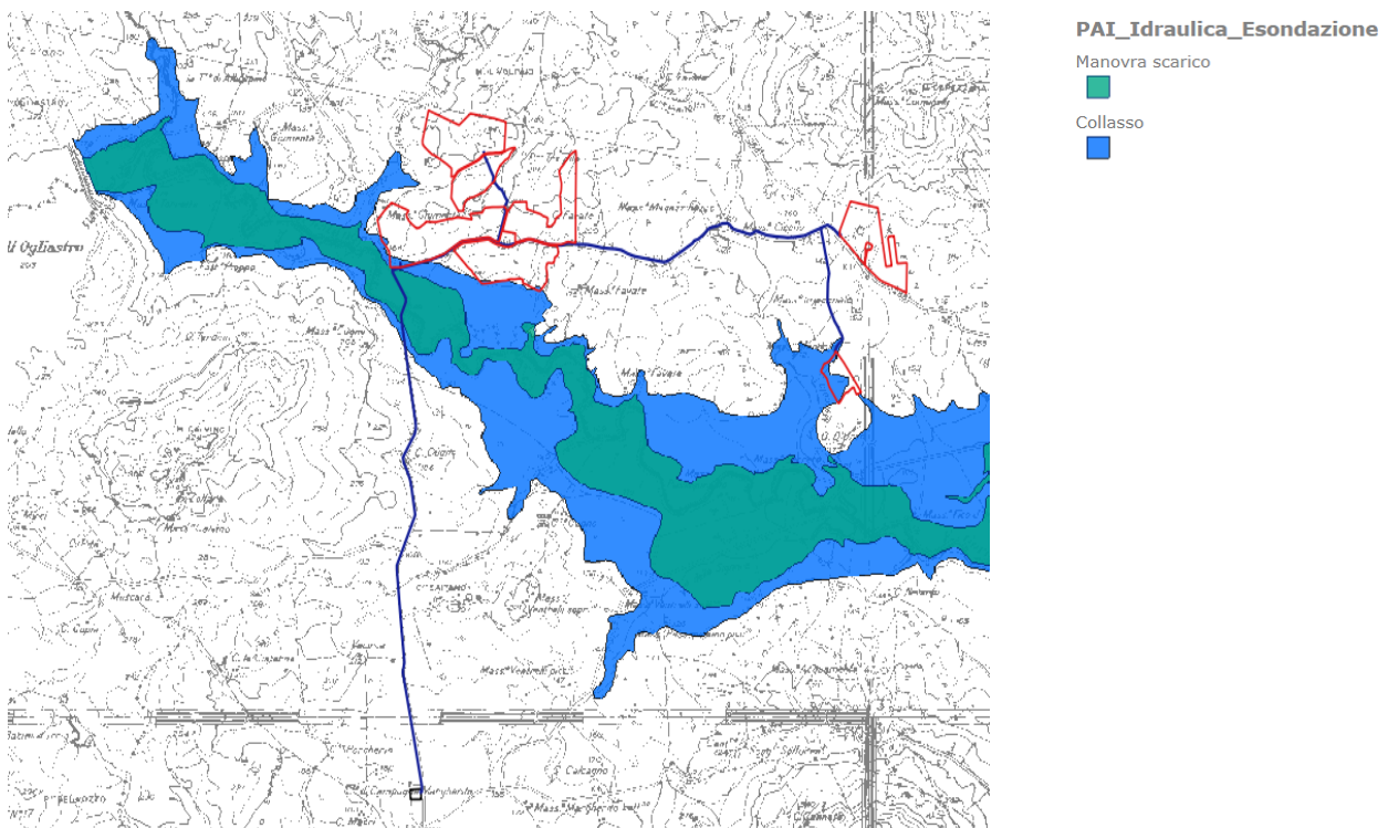
Figura 19 | Carta delle aree di esondazione per collasso e manovra degli organi di scarico della diga Ogliastro N.89 (Fonte SITR)_ In rosso le aree di progetto, in blu il cavidotto
