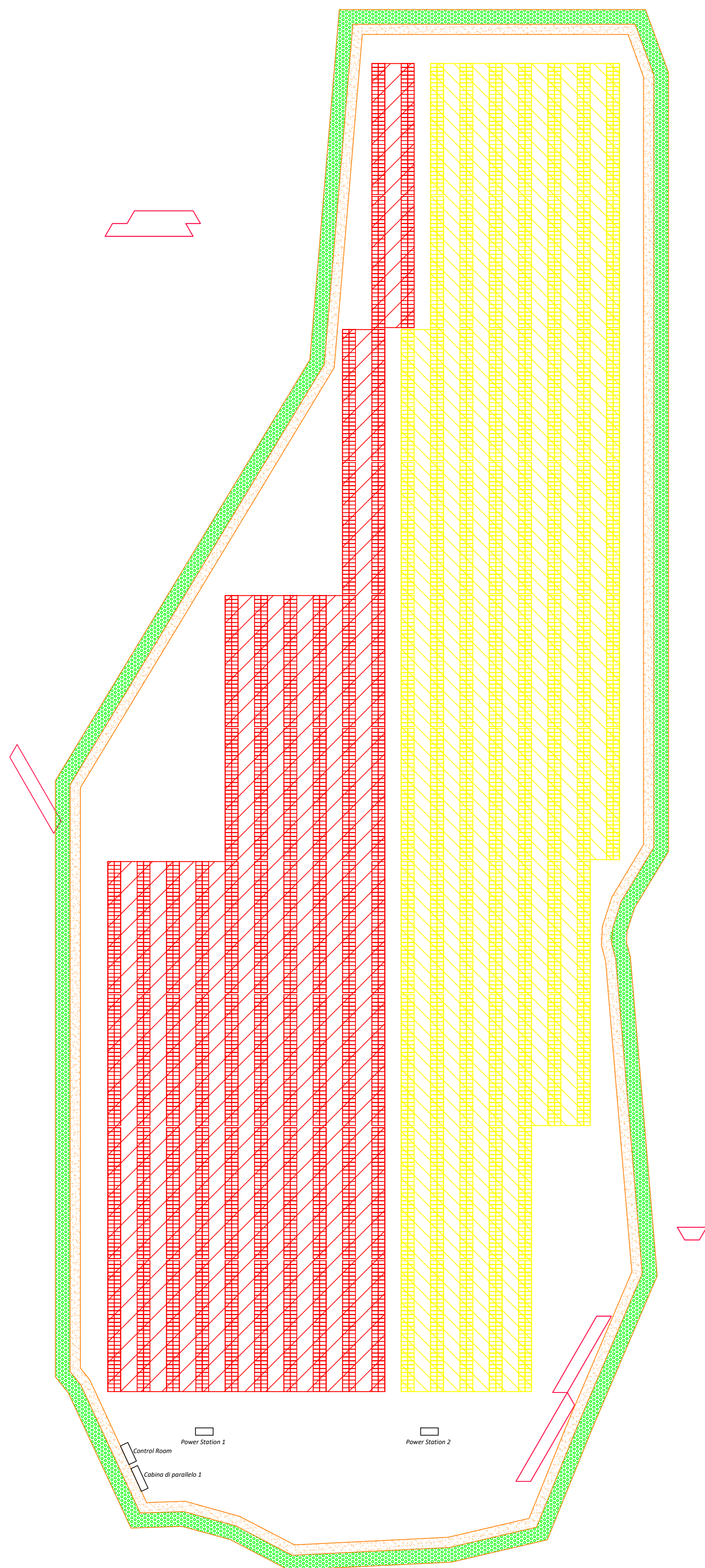
LAYOUT STRINGHE Lotto "A"
