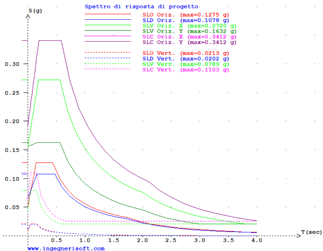
Fig. 10 - Spettri di risposta sismica di progetto - Matera
