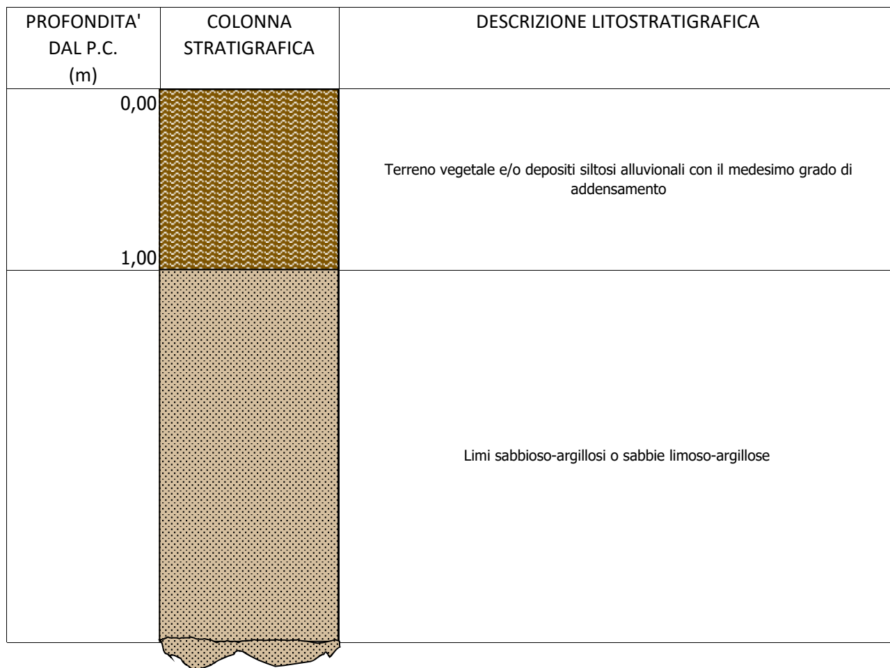
Fig.8 - COLONNA STRATIGRAFICA Realizzazione di un impianto solare fotovoltaico da 33,997 MWp Progetto "MASSERIA IESCE"
