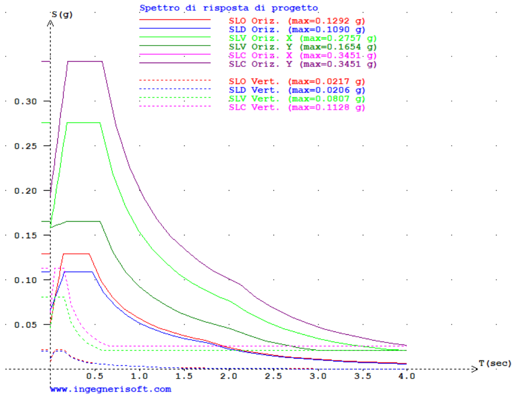
Fig. 9 - Spettri di risposta sismica di progetto - Altamura
