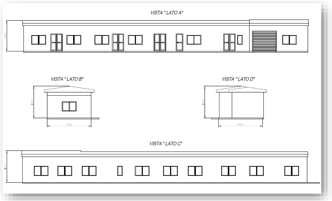
Figura 8 – Schemi grafici edificio di controllo SET
