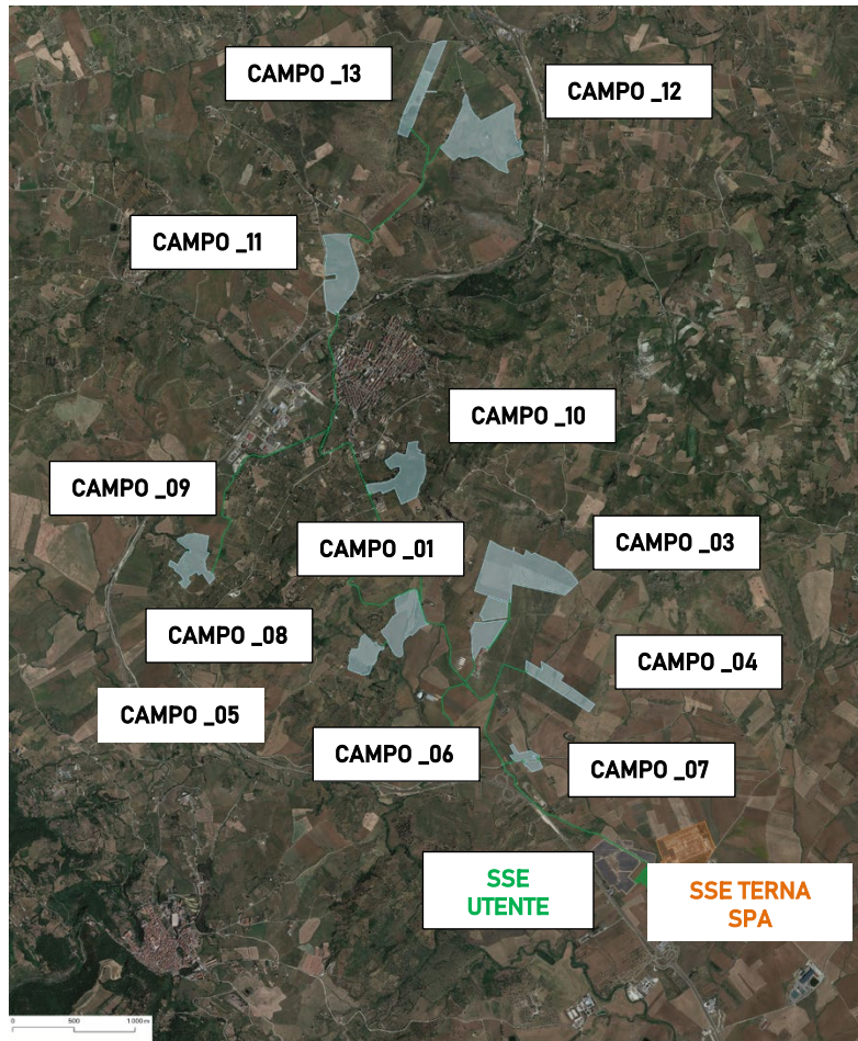
Figura 3 - Estratto Elaborato “Planimetria Impianto su Ortofoto – Stato di Fatto”
