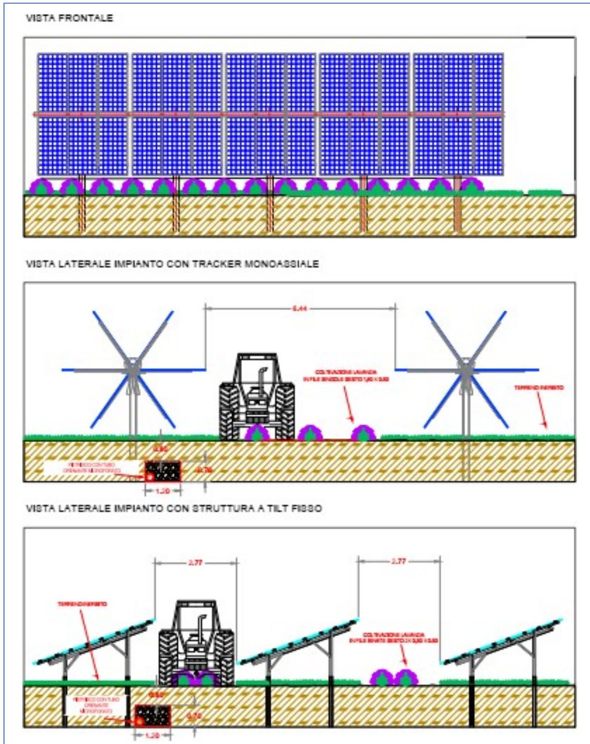
Figura 14 - Modalità di coltivazione della lavanda in funzione della tipologia di struttura di sostegno dei pannelli
