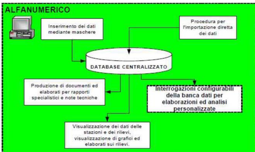
Figura 12-1 SIM Interfaccia alfanumerica
