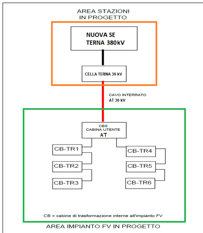
FIGURA 5: SCHEMA A BLOCCHI IMPIANTO
