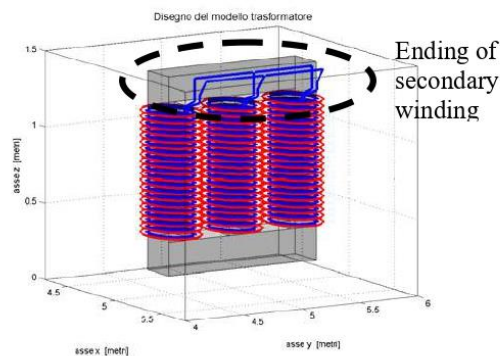
Fig. 14: Connessioni elettriche considerate al lati BT.
