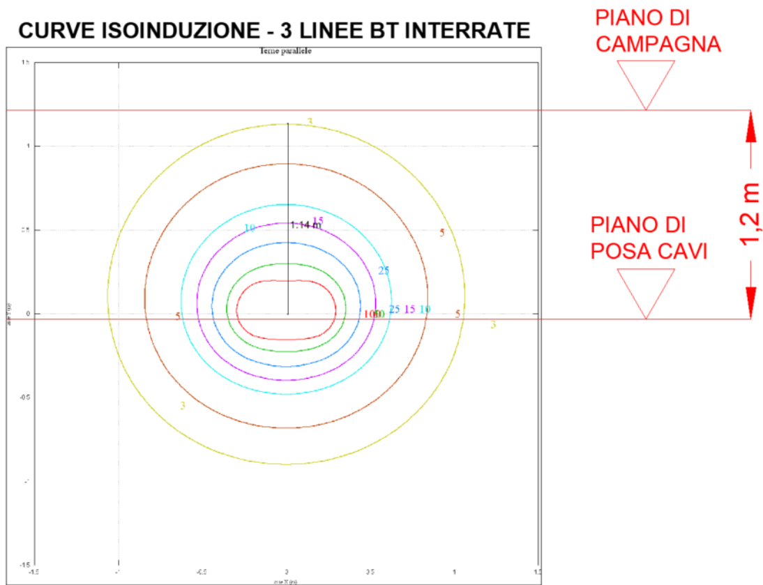
FIGURA 1: CURVE ISOINDUZIONE – 3 LINEE BT INTERRATE
