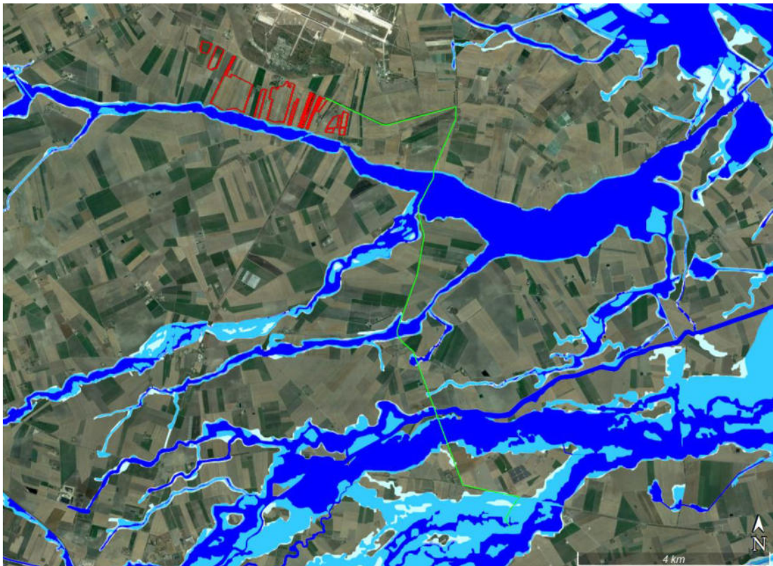
Figura 3.14: Stralcio assetto idrogeologico (PAI) - assetto idraulico territorio ex Autorità di Bacino della Puglia pubblicato sulla gazzetta ufficiale del G.U. n. 194 del 20/08/2019. In verde la linea di connessione alla RTN, in rosso il sito di progetto.
