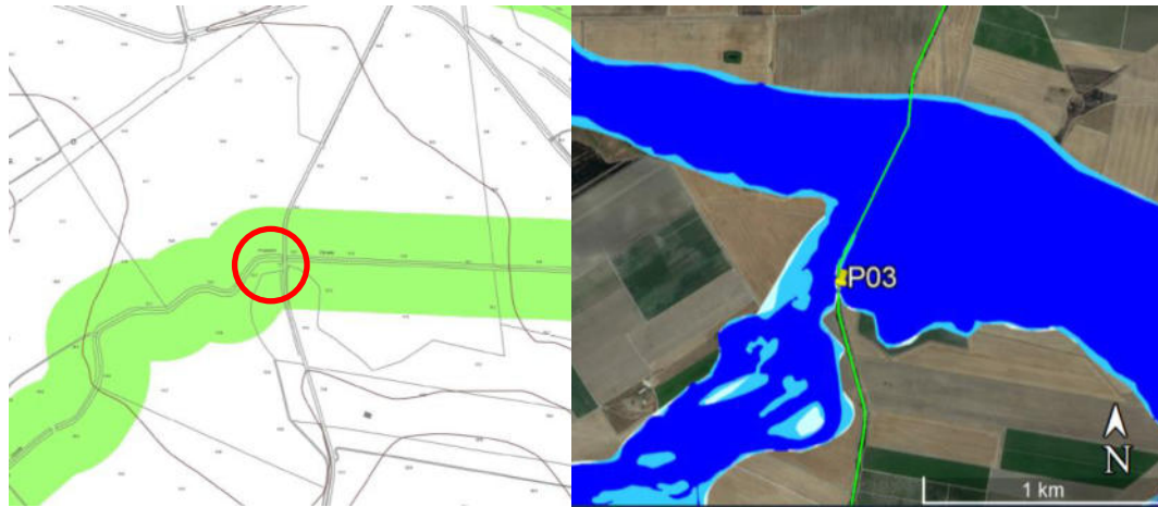
Figura 5.12: A sinistra stralcio del PGRA con in verde la fascia fluviale del canale Properzio. A destra stralcio del PAI con fasce di pericolosità idraulica Alta, Media e Bassa.
