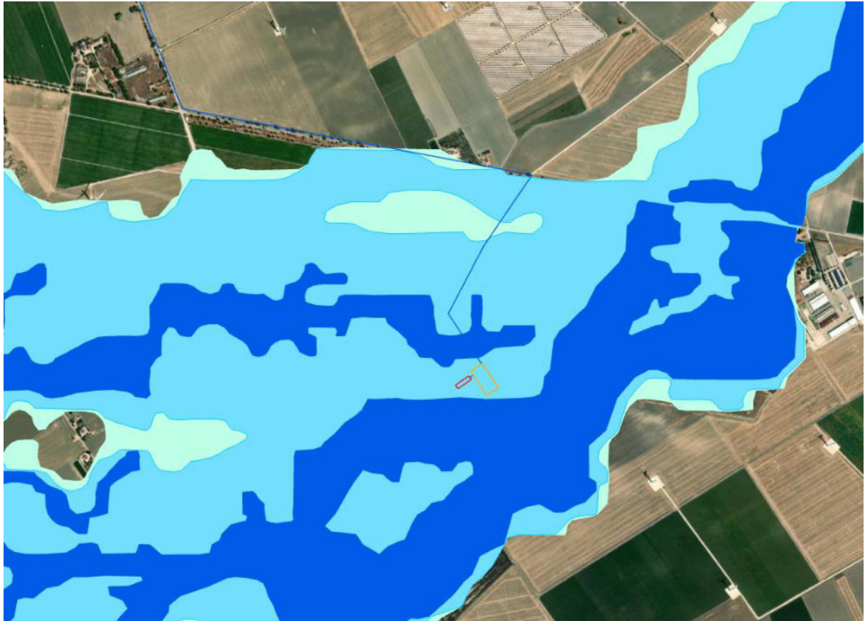
Figura 5.32: Stralcio del pgra secondo ciclo con relative fasce di pericolosità media e bassa e blu la linea di connessione. In arancione la cabina in esame.
