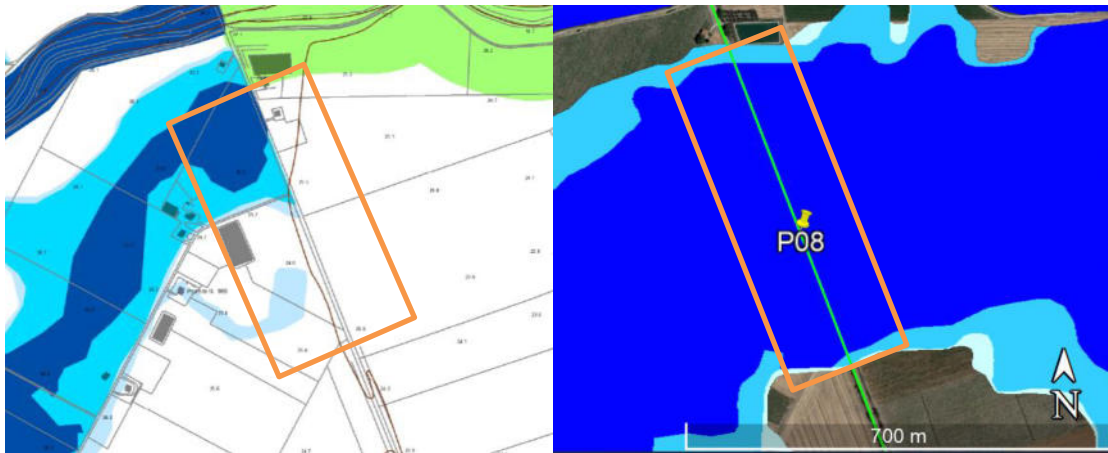
Figura 5.23: A sinistra stralcio del PGRA con in rosso l'area di interferenza. A destra stralcio del PAI con relative fasce di pericolosità idraulica e in verde. In arancione il tratto in esame.
