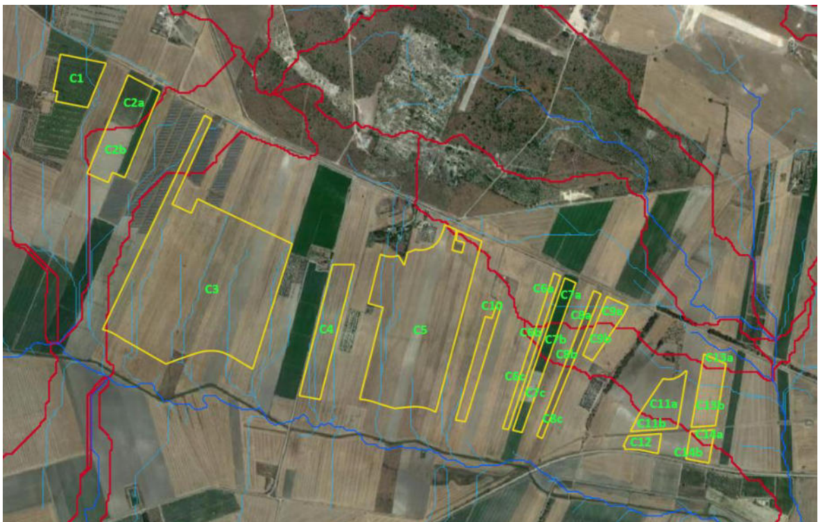
Figura 6.5: Delimitazione bacini scolanti e codifica (giallo), reticolo di drenaggio esterno ed interno alle sezioni di progetto (blu) e limiti dei bacini idrografici (rosso).
