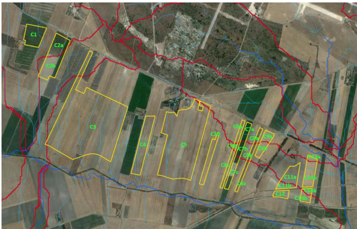
Figura 6.9: Delimitazione aree di impianto e rete di drenaggio naturale interna.
