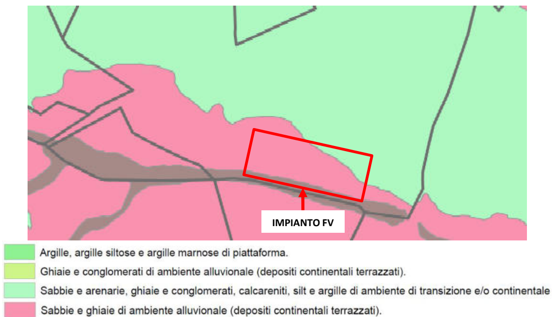
Figura 6.6: Stralcio carta geolitologica (Fonte: AdBP Candelaroe - Allegato 1.2.1). In rosso l'area di progetto.
