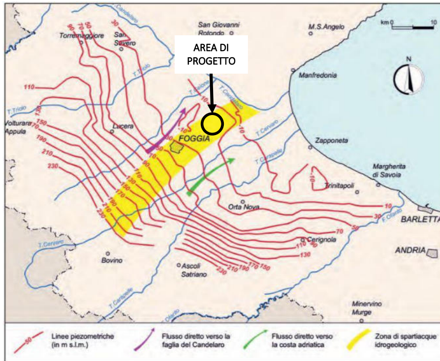
Figura 3.7: Isopieziche della falda superficiale del Tavoliere relativa all'anno 2003 con indicazione delle zone ove è ubicato lo spartiacque idrogeologico (fonte ISPRA). In evidenza, l'area di progetto.
