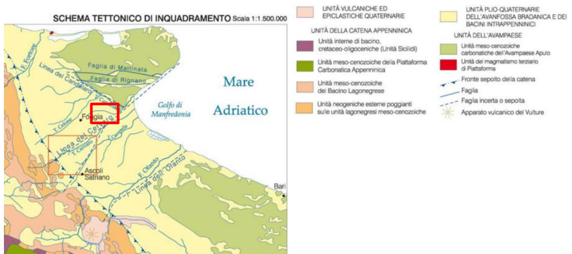
Figura 3.4: Schema geologico e strutturale dell'area del Tavoliere e del Subappennino Dauno
