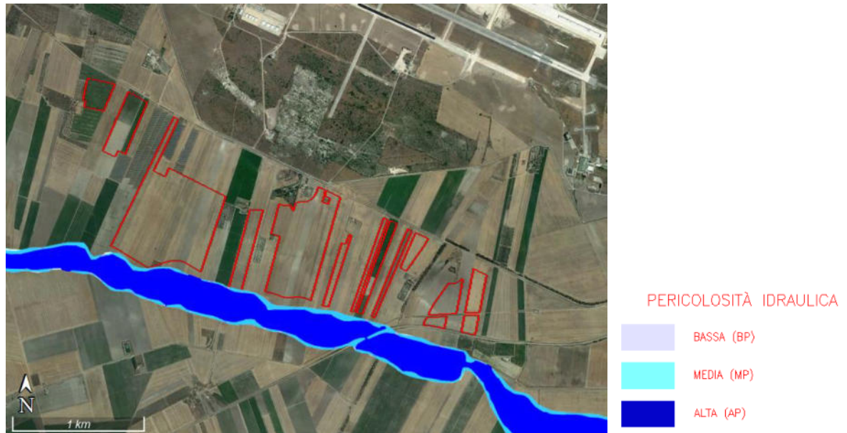
Figura 3.12: Stralcio assetto idrogeologico (PAI) - assetto idraulico territorio ex Autorità di Bacino della Puglia pubblicato sulla gazzetta ufficiale del G.U. n. 194 del 20/08/2019. In rosso il sito di progetto.
