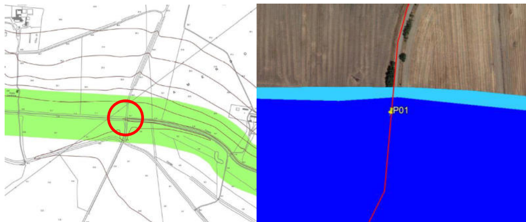
Figura 5.6: A sinistra stralcio del PGRA con in verde la fascia fluviale del C. Farano. A destra stralcio del PAI con fasce di pericolosità idraulica Alta e Media.
