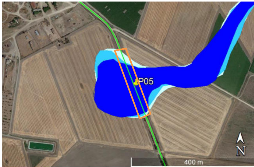
Figura 5.16: Stralcio PAI 2019 con fasce di pericolosità alta, media e bassa e in verde la linea di connessione. Interferenza P05. In arancione il tratto in esame.
