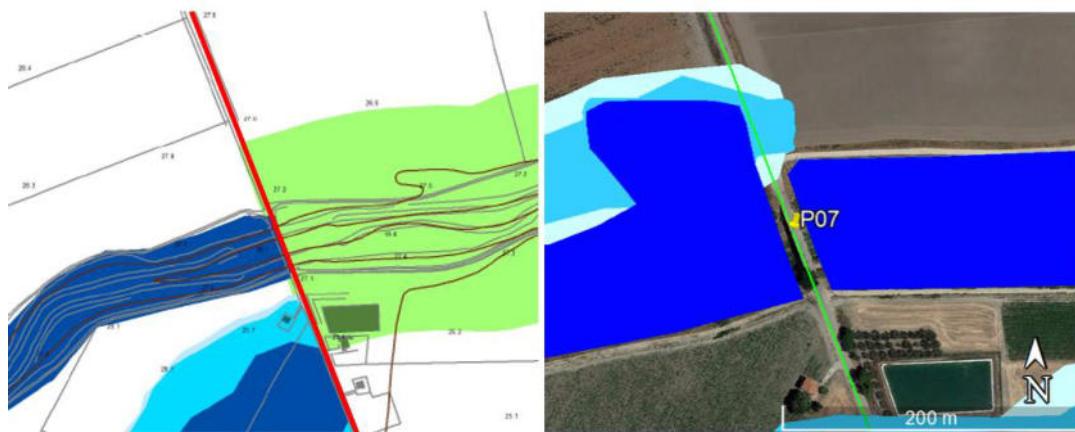
Figura 5.21: A sinistra stralcio del PGRA con in rosso la linea di connessione e area di pericolosità alta. A destra stralcio del PAI con relative fasce di pericolosità e linea di connessione in verde.
