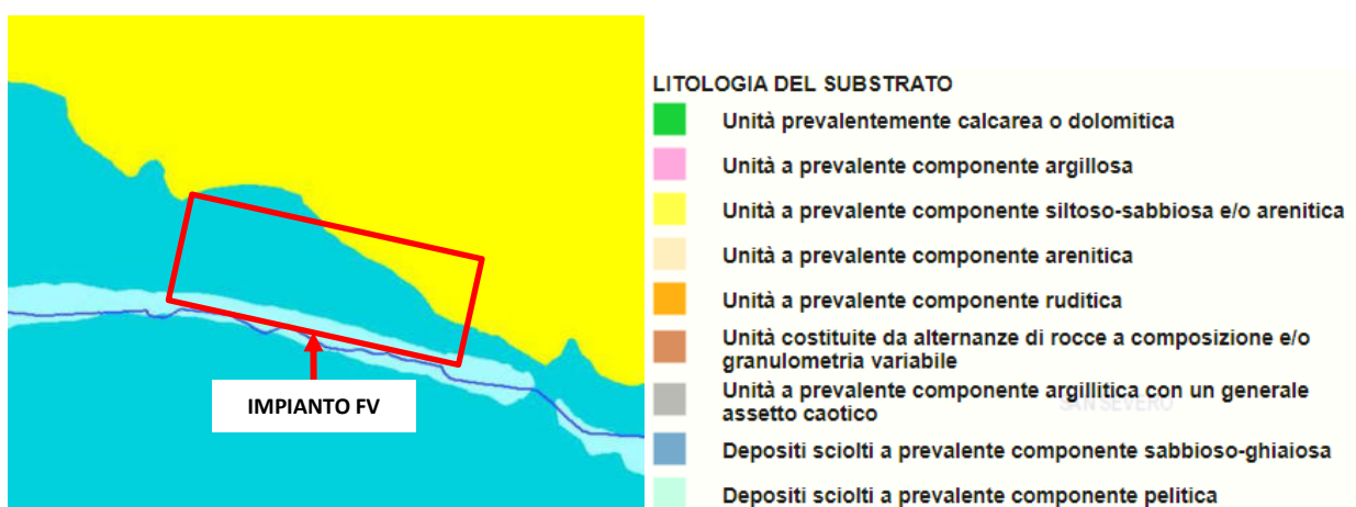
Figura 3.11: Stralcio carta idrogeomorfologica della Regione Puglia aggiornata al 21/02/2017.
