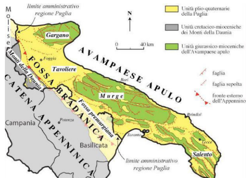
Figura 3.3: Carta geologica schematica della regione Puglia (da Pieri et al. 1997, modificata).
