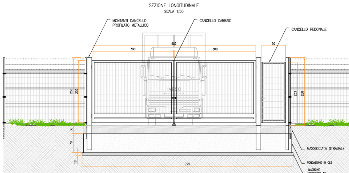
Figura 4.7: Particolare accesso
