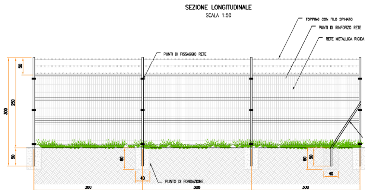
Figura 4.5: Particolare recinzione
