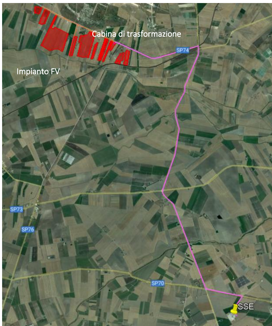
Figura 4.8: In magenta il percorso di connessione dal campo FV alla SSE
