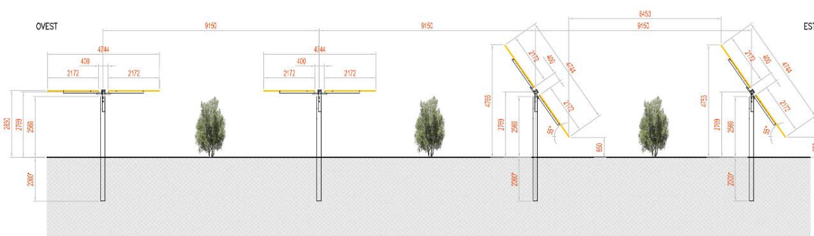
Figura 6.4: Tipologico – Vista in Sezione dell'impianto Olivicolo
