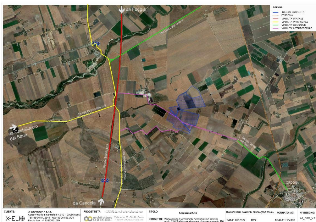
AS_ORD_V.17 - sistema viario di accesso al sito
