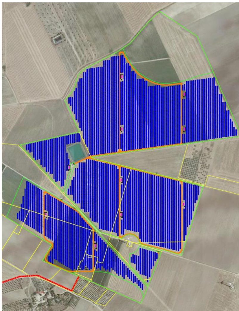
Layout dell'area di intervento
