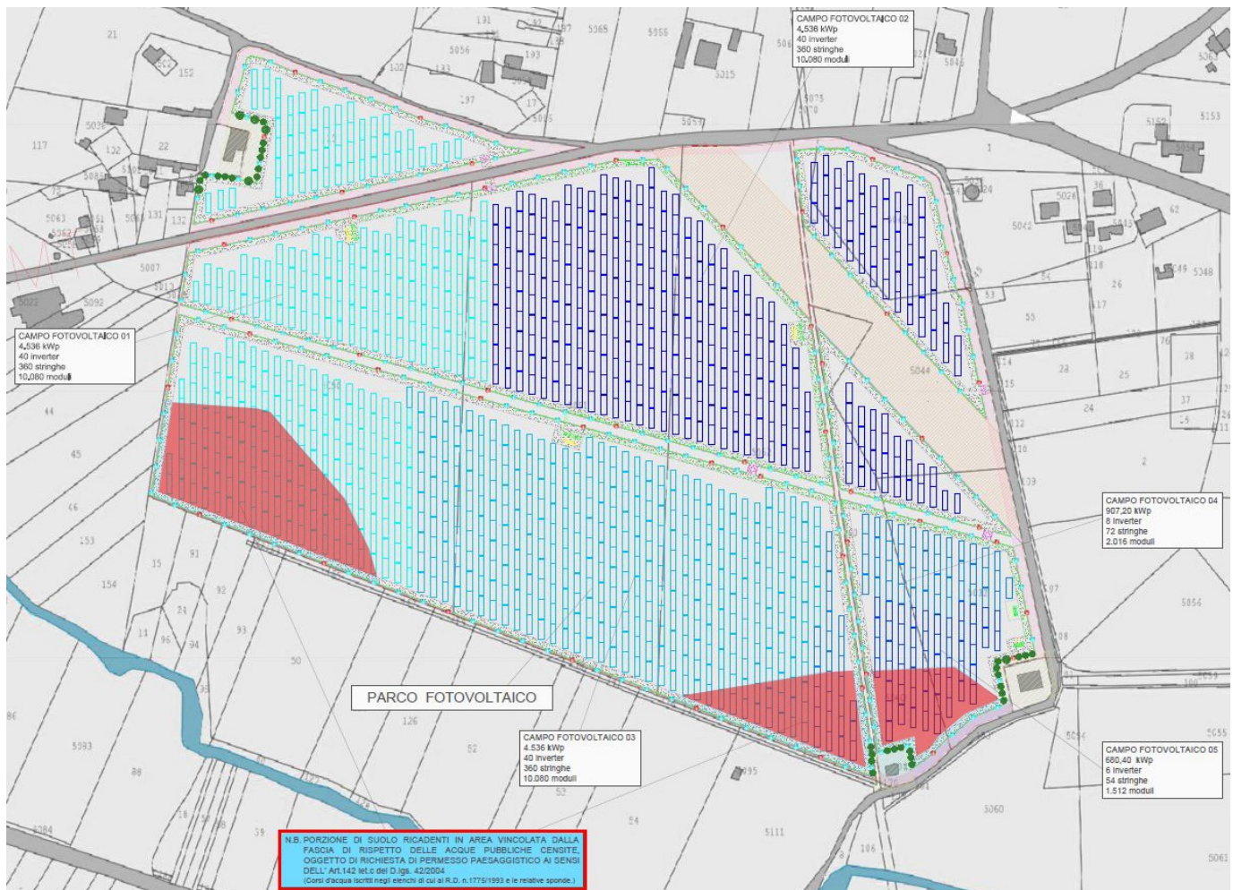
Stralcio Layout di Progetto con aree ricadenti nella fascia di rispetto del "Rio Travata"
