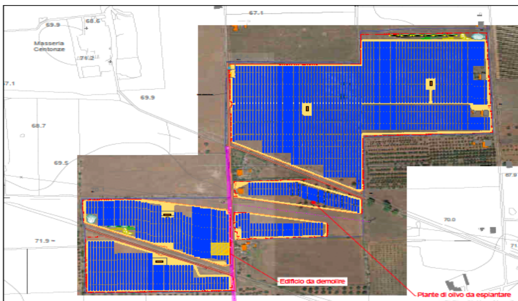
Tavola n. 1: Impianto suddiviso in campi e sottocampi fotovoltaici.
