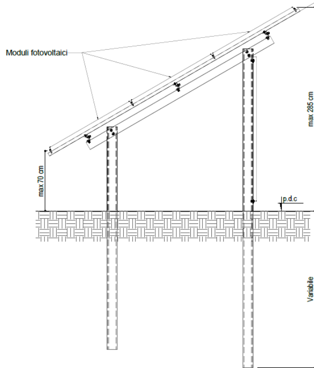
Figura 9 - Sezione pannello fotovoltaico su supporto
