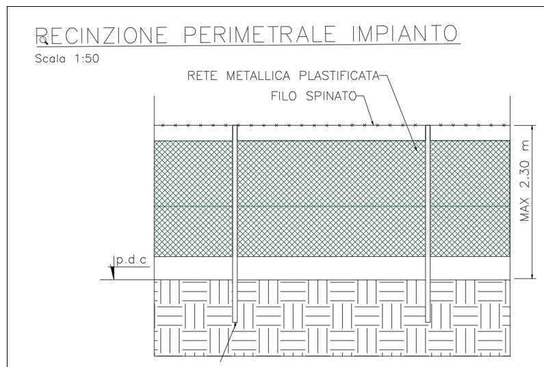
Figura 13 - Tipico recinzione perimetrale area impianto di generazione
