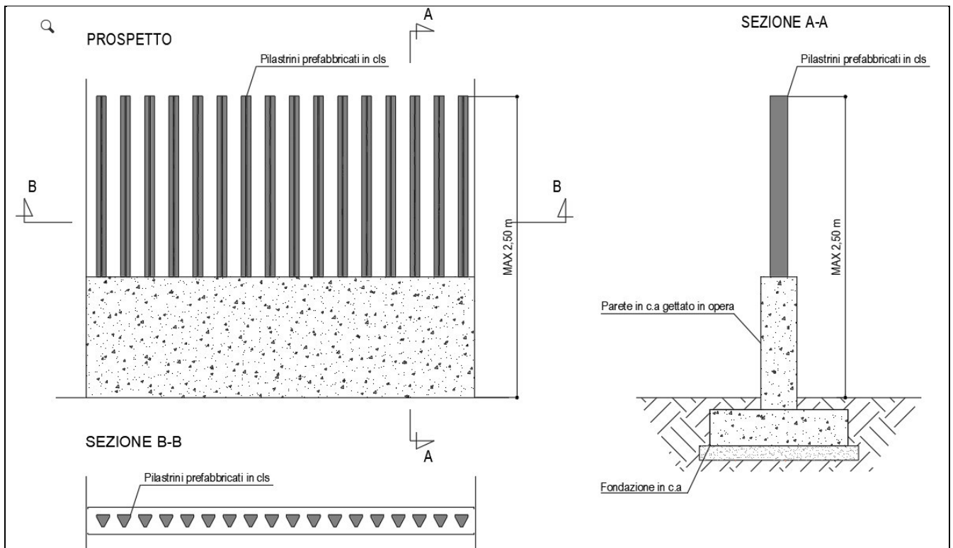
Figura 14 - Tipico recinzione perimetrale SE utente ed impianto di generazione
