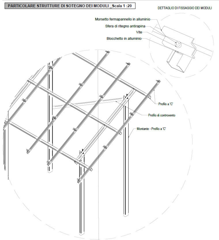
Figura 10 – Stralcio Particolare costruttivo supporto
