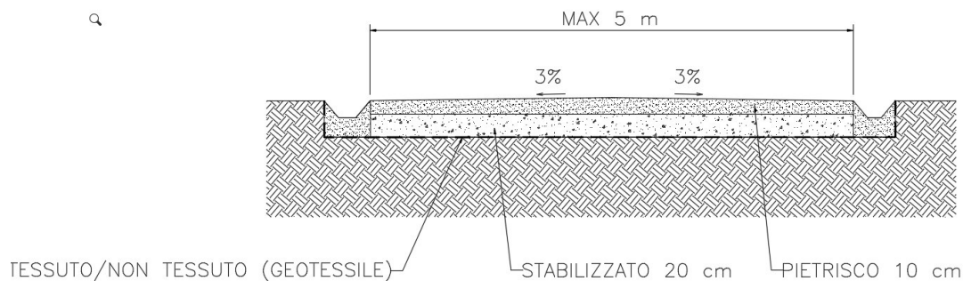
Figura 11 - Sezione tipo -viabilità interna
