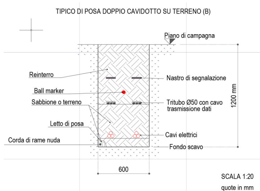
Figura 12 - Tipico posa cavidotto su terreno
