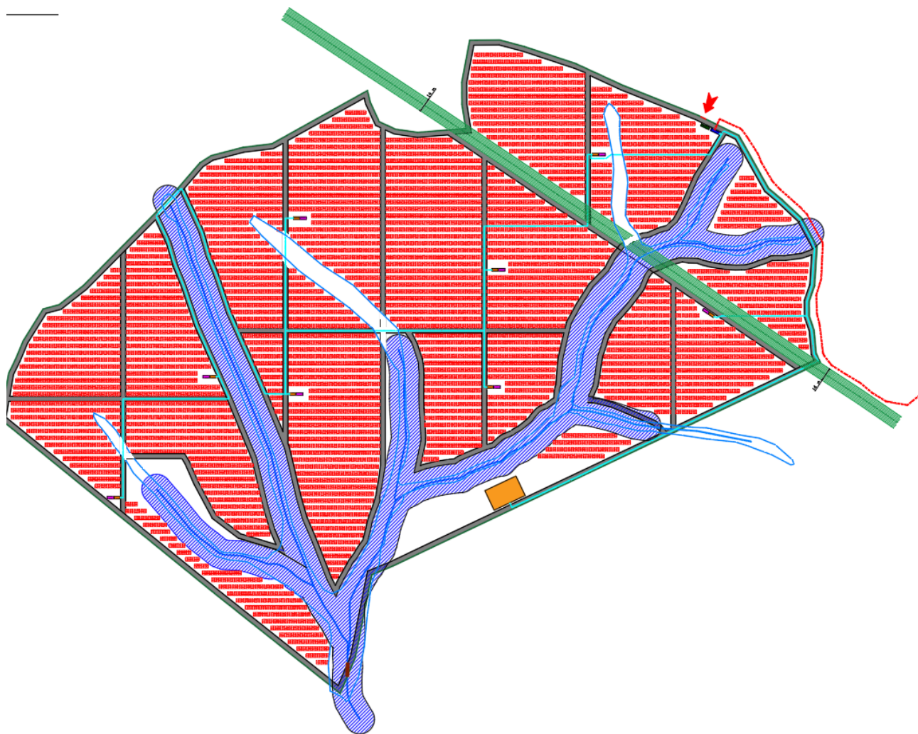
Figura 5 - Stralcio Layout impianto
