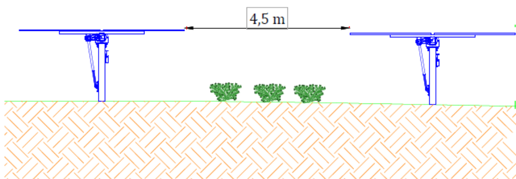
Schema coltivazione agro-voltaico
