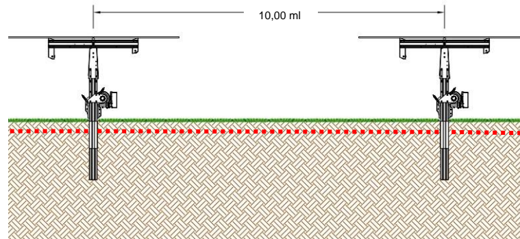
Figura 8 – Distanza tra le singole file (tracker) di moduli fotovoltaici con indicazione della superficie che può essere utilizzata per la messa a coltura di prato stabile e lavandeto (linea tratteggiata rossa).
