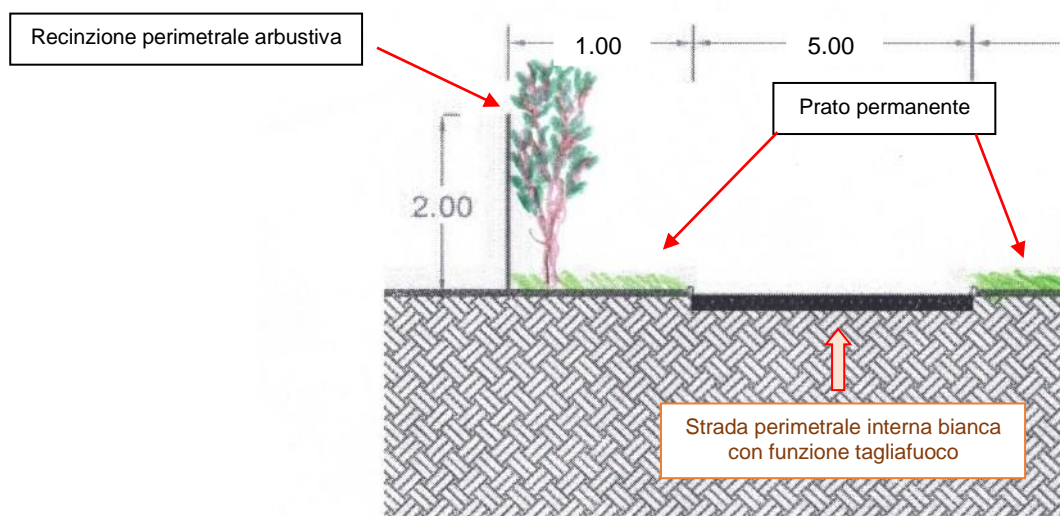
Figura 14 – Sezione tipo d’impianto della siepe
