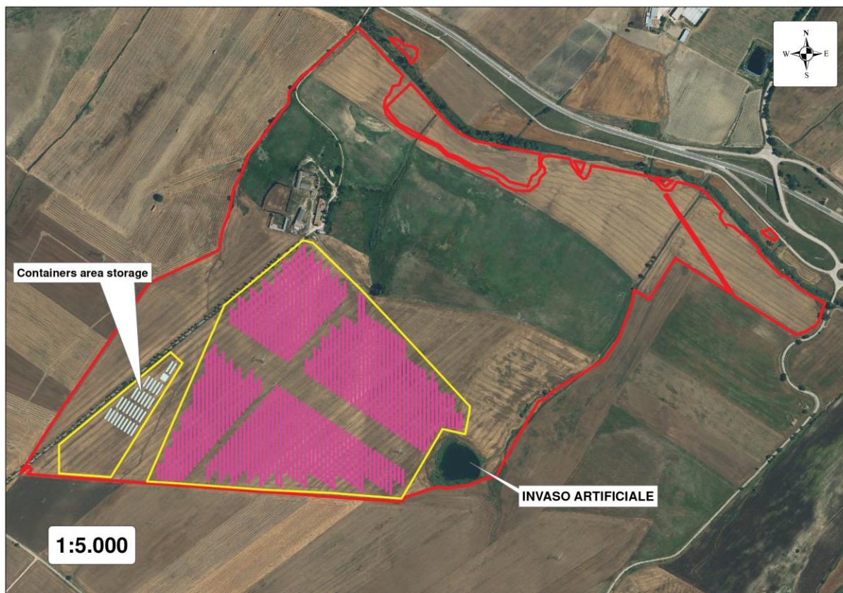
Figura 7 – Area di pertinenza del progetto con indicazione dell’ubicazione dei pannelli fotovoltaici, dei containers dell’area “storage” e della recinzione perimetrale.
