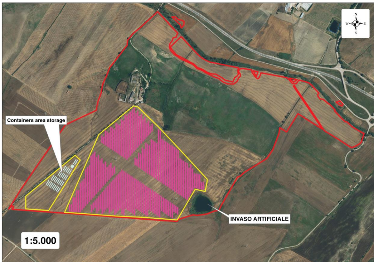
Figura 4 – Area di pertinenza del progetto con indicazione dell’ubicazione dei pannelli fotovoltaici, dell’area storage e della recinzione perimetrale.
