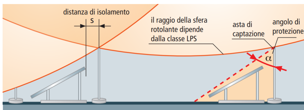
Metodo della sfera rotolante
