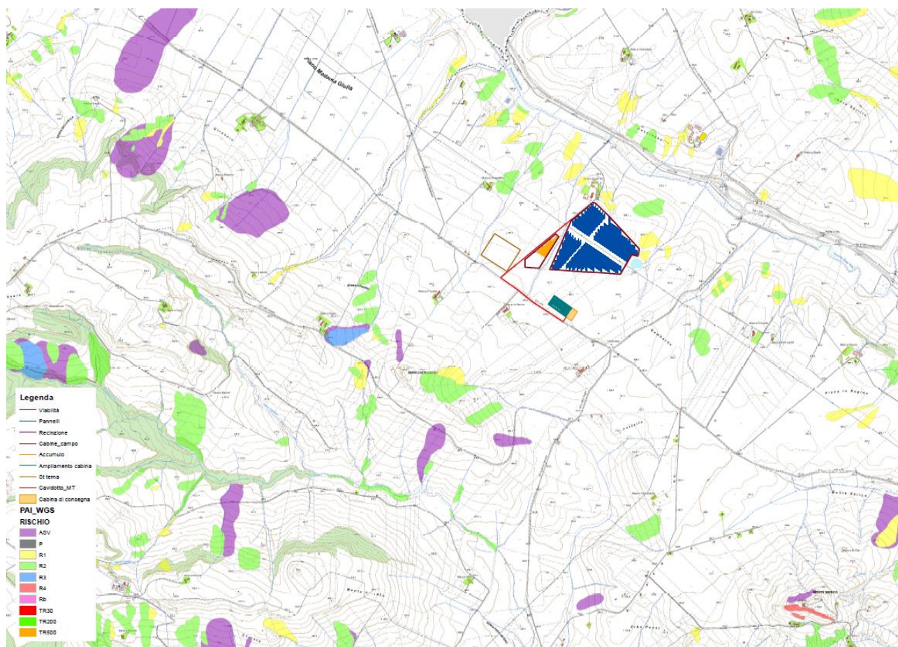
Figura 3.2. – Stralcio Carta delle Frane: localizzazione impianto.
