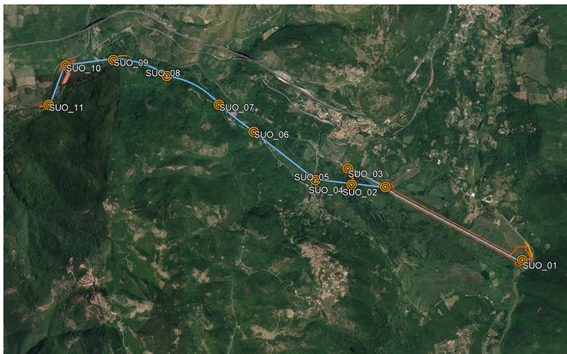
Figura 7-1 Ubicazione dei punti di monitoraggio della componente suolo
