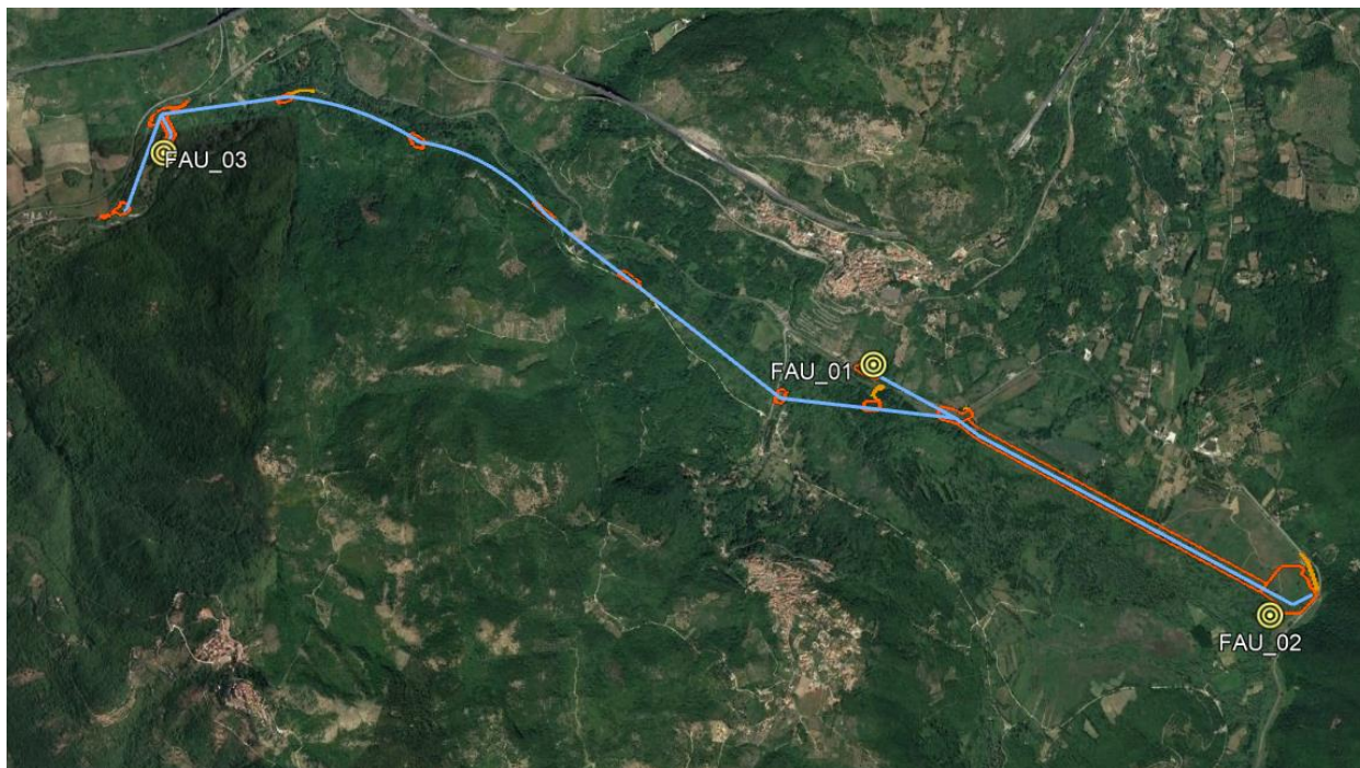
Figura 9-1 Localizzazione punti di monitoraggio su ortofoto. In blu il tracciato di progetto
