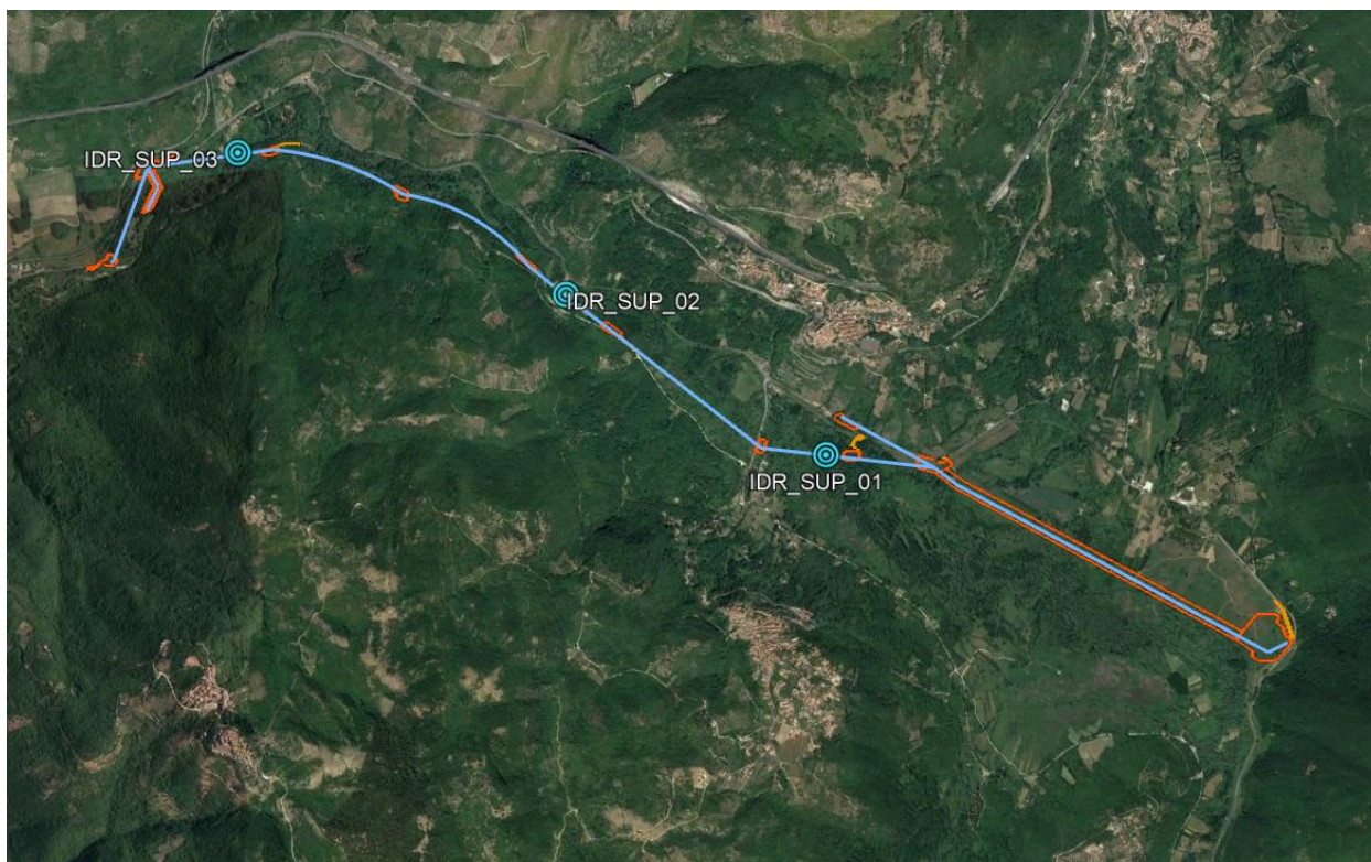
Figura 5-1 Ubicazione dei punti di monitoraggio delle acque superficiali
