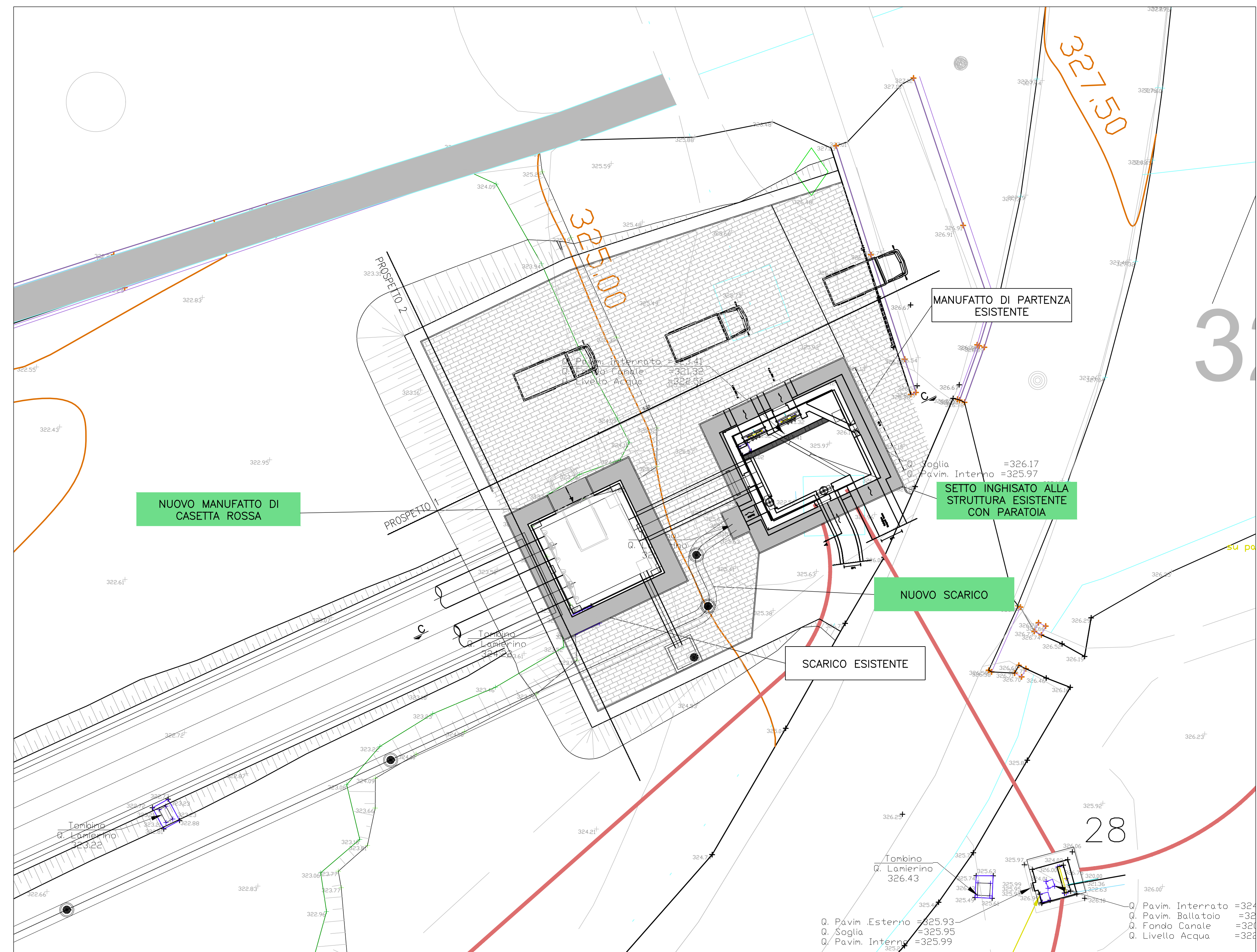
STRALCIO PLANIMETRICO NUOVO MANUFATTO DI PARTENZA - SCALA 1:200
