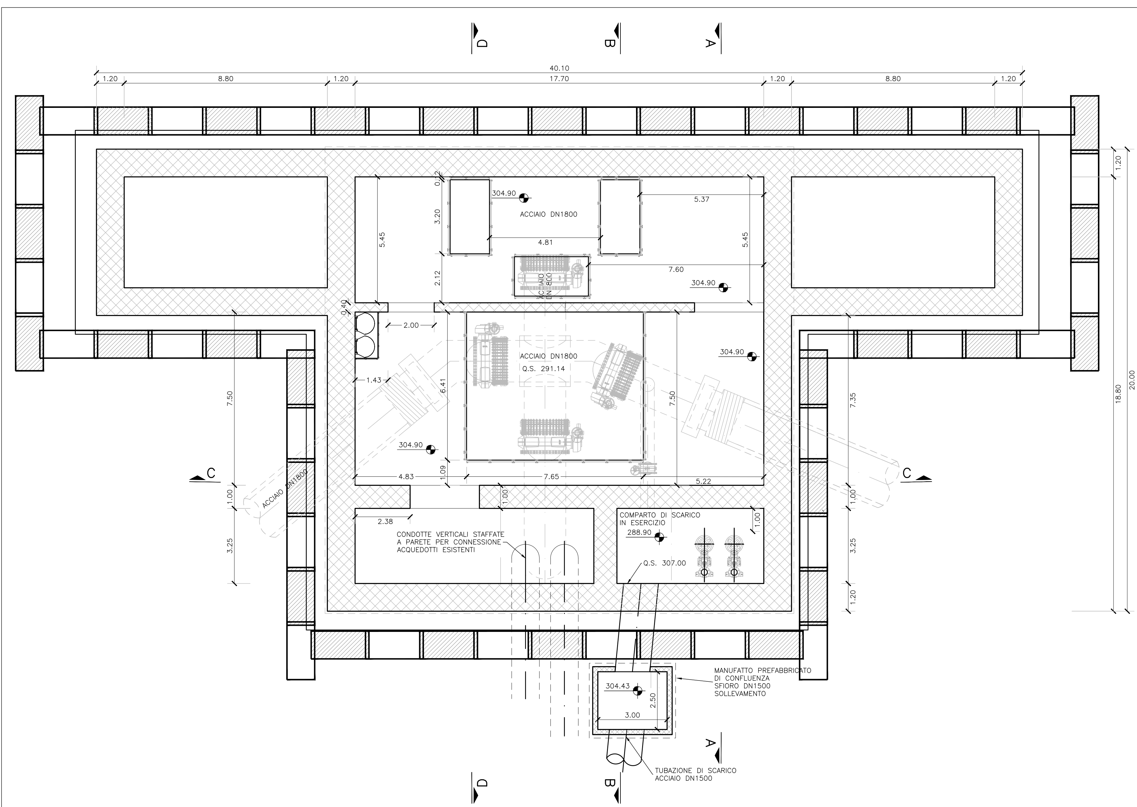
PIANTA P2 MANUFATTO INTERCONNESSIONE (P27) SCALA 1:100
