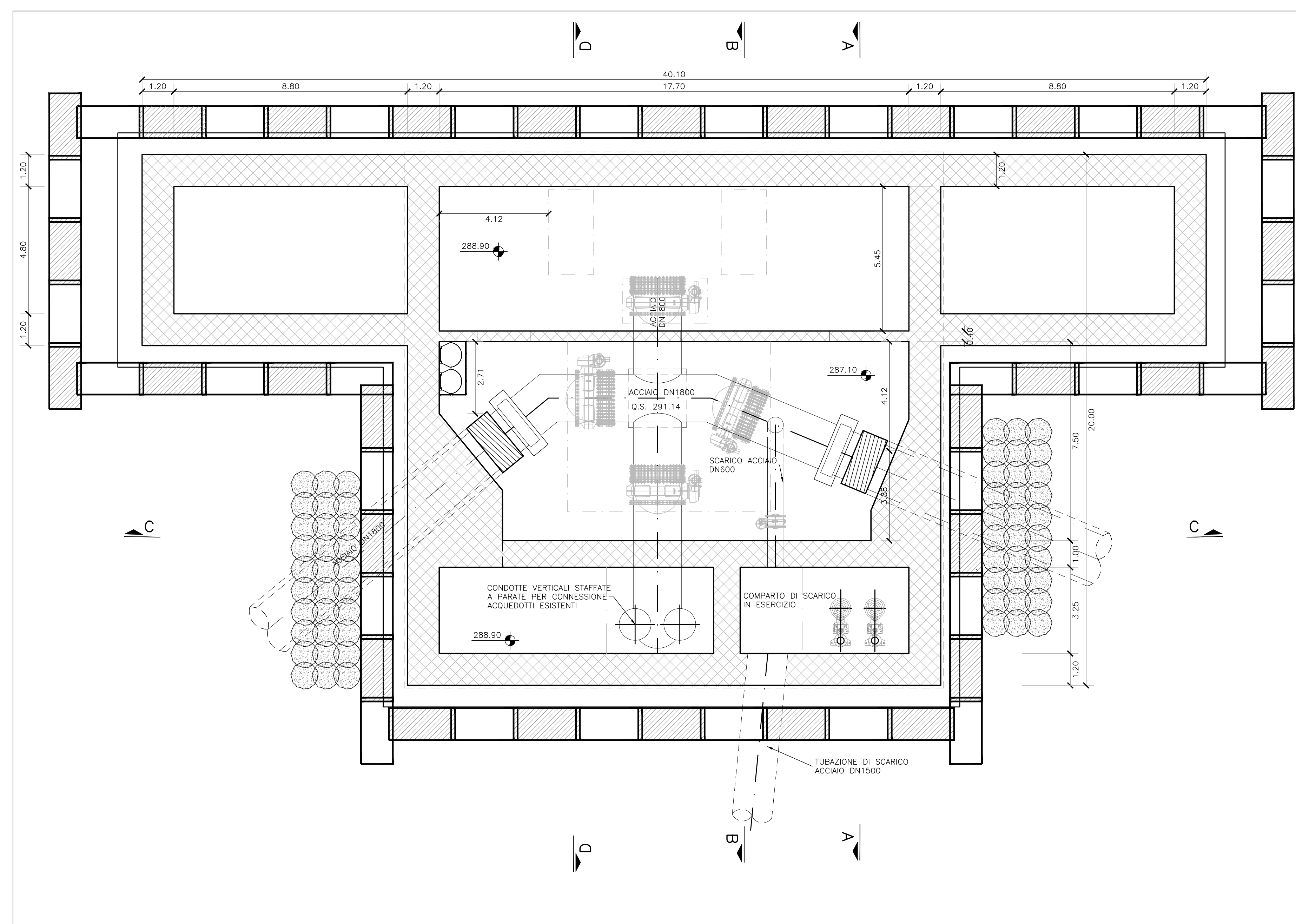
PIANTA P3 MANUFATTO INTERCONNESSIONE (P27) SCALA 1:100
