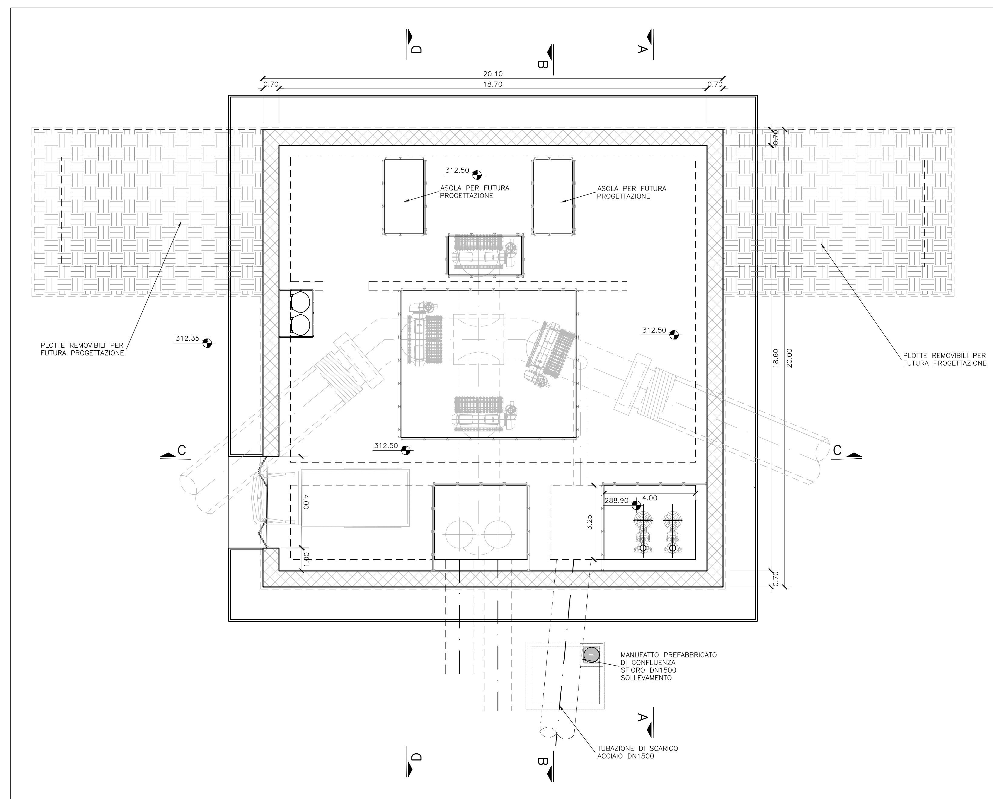
PIANTA P1 MANUFATTO INTERCONNESSIONE (P27) SCALA 1:100
