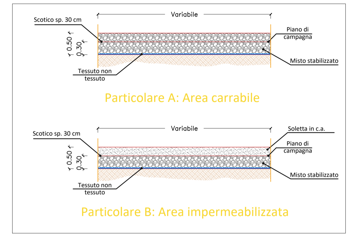
PARTICOLARI SCALA 1:50
