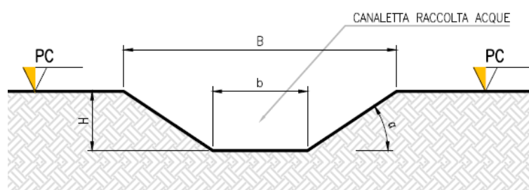
Figura 5.2: Sezione tipologica cunetta di drenaggio realizzata in scavo
