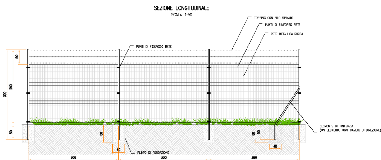
Figura 5.1 Tipo recinzione
