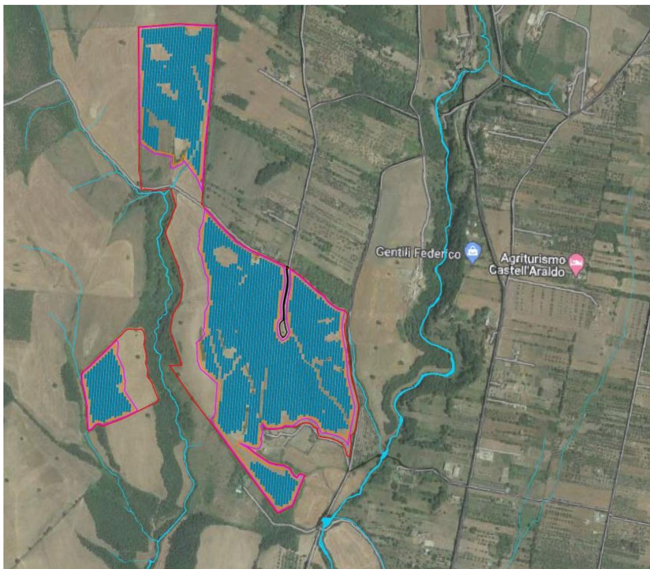
Figura 3: Layout preliminare di impianto
