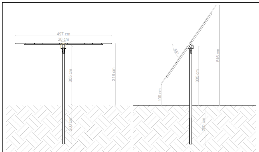
FIGURA 2: SCHEMA TIPO TRACKER AD ASSE VARIABILE
