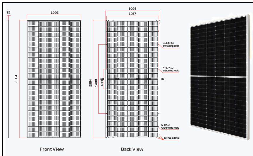
FIGURA 1: PANNELLO FV PARI A 550 WP – IN CONDIZIONI STANDARD - CON DIMENSIONI 2384 X 1096 X 35 MM
