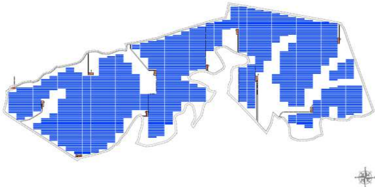
Figura 39. Layout dell'impianto
