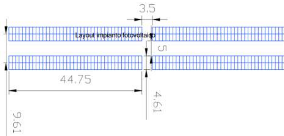
Figura 38. Distanze trackers
