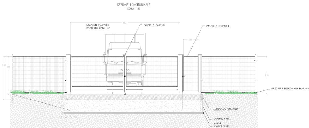
Figura 5.2: Particolare accesso
