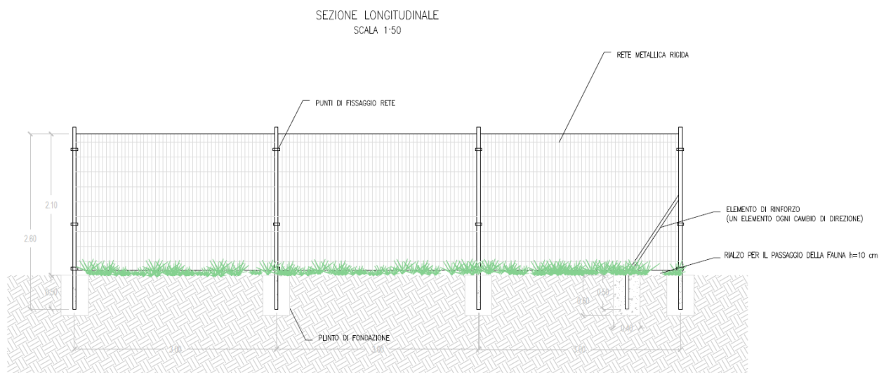
Figura 5.1: Particolare recinzione
