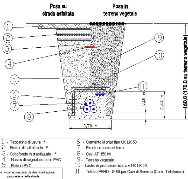
Figura 3: Tipici di posa cavo AT con n°1 linea su viabilità asfaltata e sterrata
