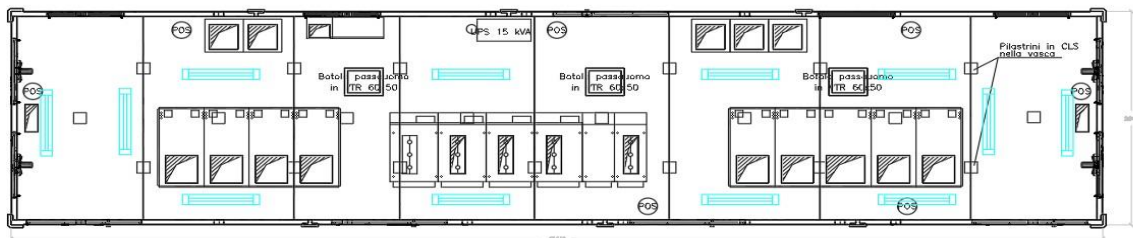
Figura 4.4 - Posizionamento plafoniere Cabina Power Station - cabina BT/MT.
