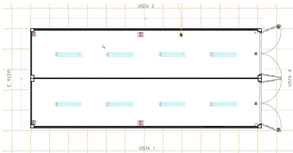
Figura 4.2 - Posizionamento plafoniere Magazzino.
