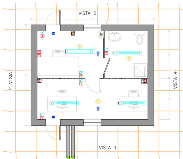
Figura 4.3 - Posizionamento plafoniere Cabina Uffici.
