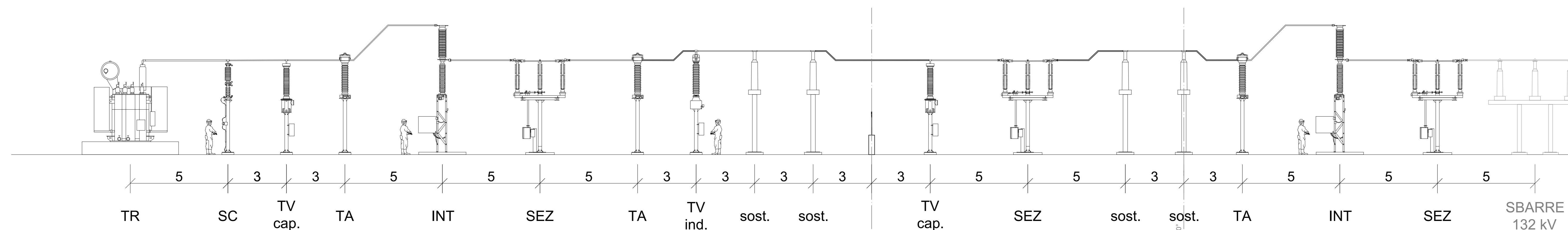
PROFILO LONGITUDINALE - scala 1:100
