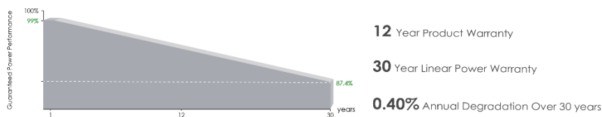
Figura 4.1 - Modulo fotovoltaico tipo: JKM595-615N-78HL4-(V)
