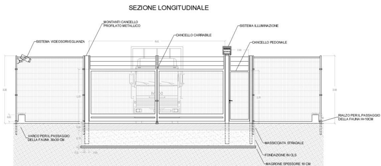
Figura 5.1: Tipico recinzione
