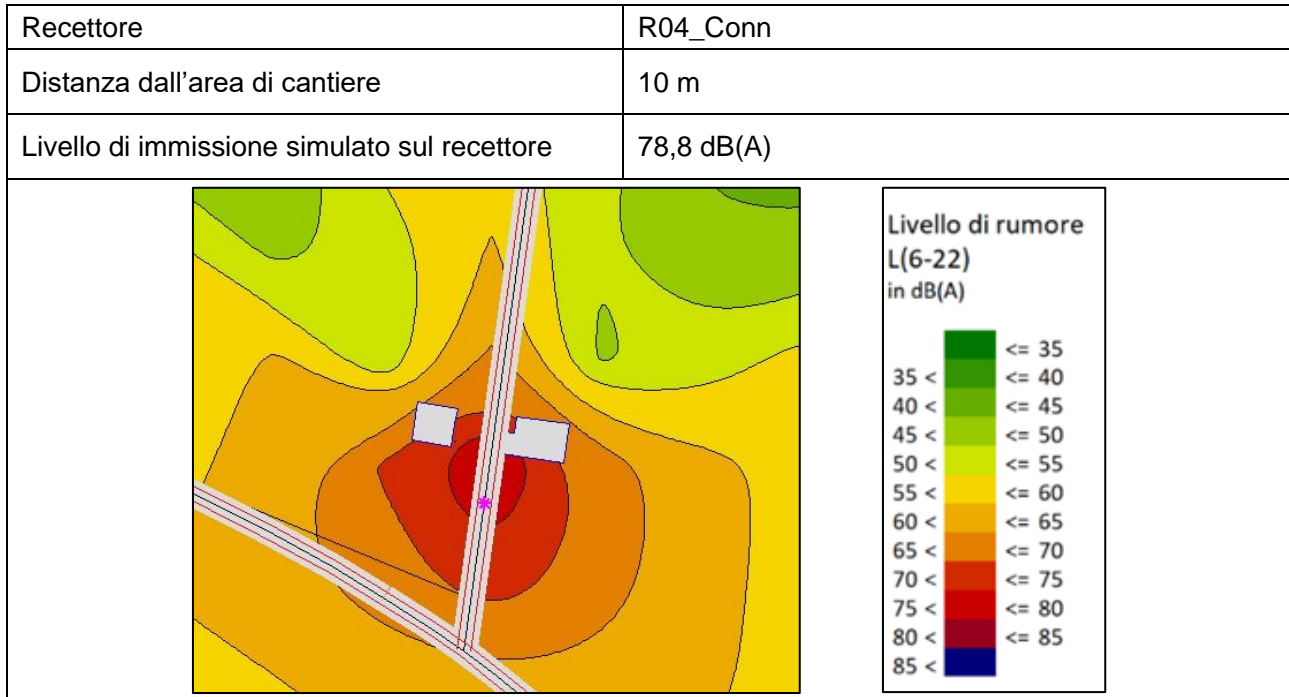
Figura 8.10 – Riepilogo simulazione – Ricettore R04_CONN
