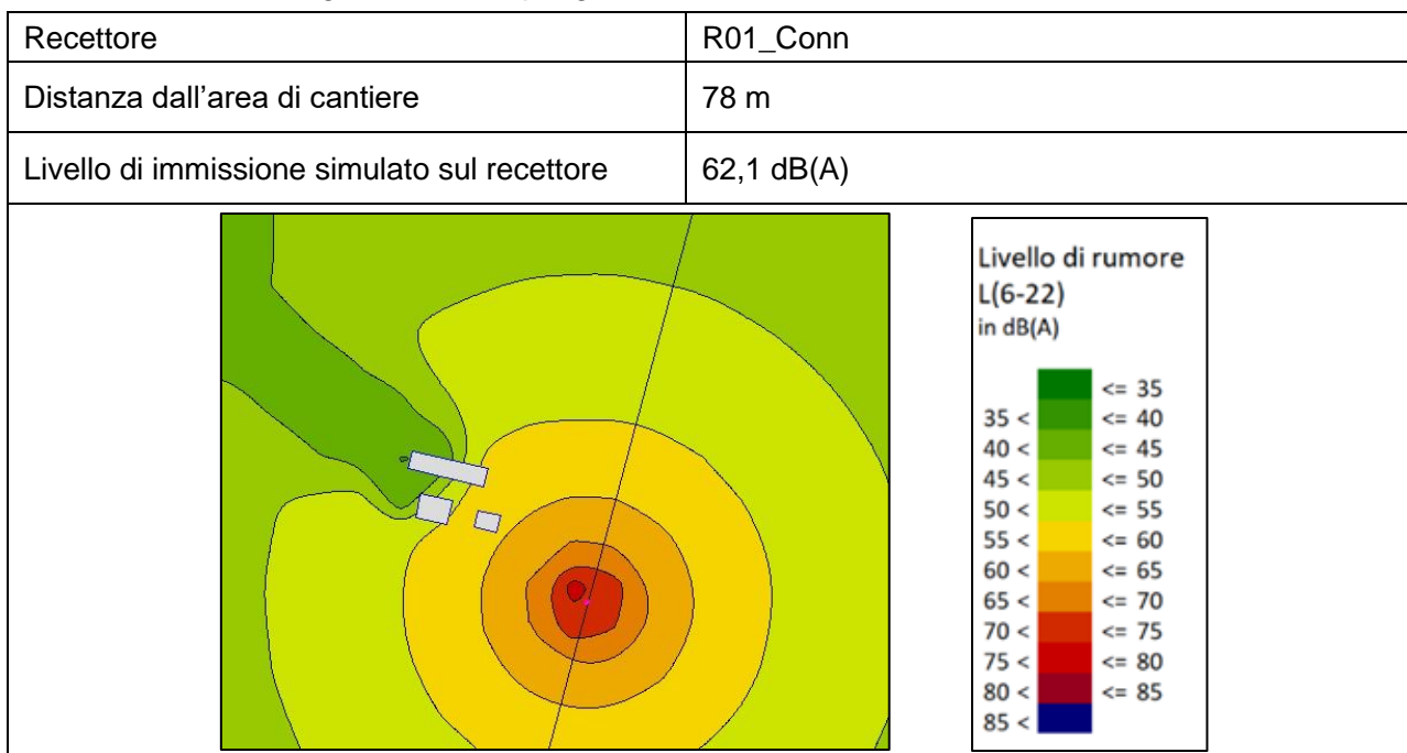
Figura 8.7 – Riepilogo simulazione – Ricettore R01_CONN
