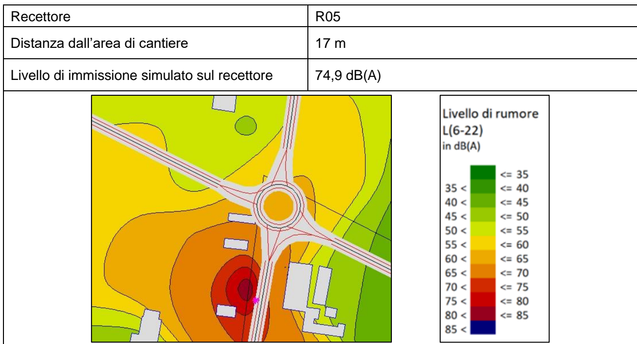
Figura 8.11 – Riepilogo simulazione – Ricettore R05
