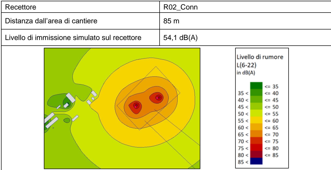
Figura 8.8 – Riepilogo simulazione – Ricettore R02_CONN
