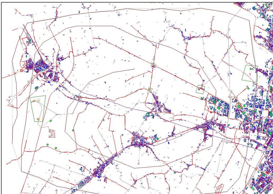
Figura 8.2 – Modello acustico dell'area di studio in SoundPlan
