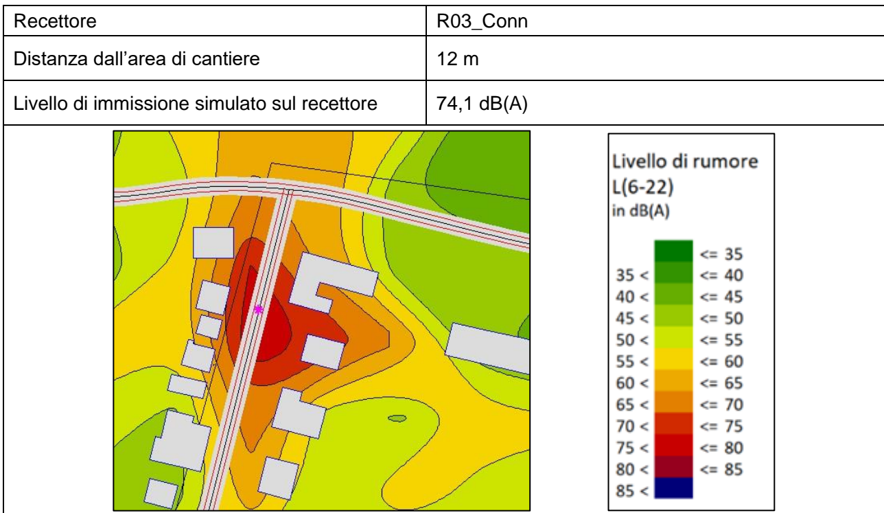
Figura 8.9 – Riepilogo simulazione – Ricettore R03_CONN
