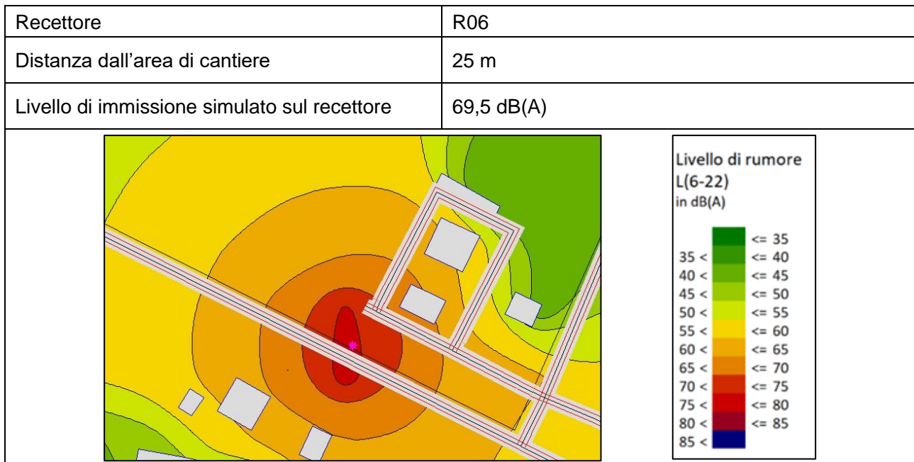
Figura 8.12 – Riepilogo simulazione – Ricettore R06
