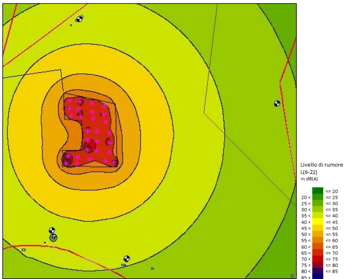
Figura 8.6 – Immagine rappresentante curve di isolivello
