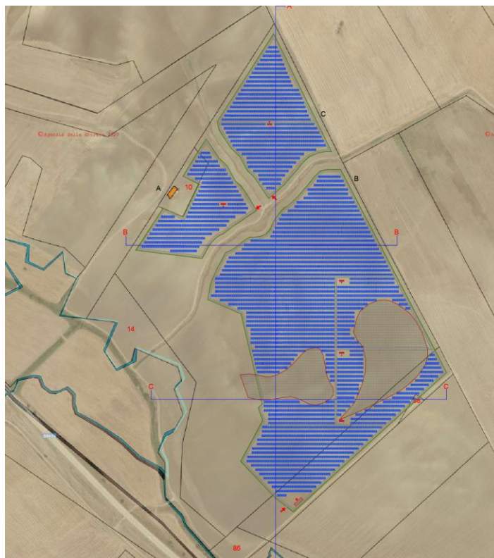
Planimetria generale impianto fotovoltaico (stralcio dalle tavole di progetto)
