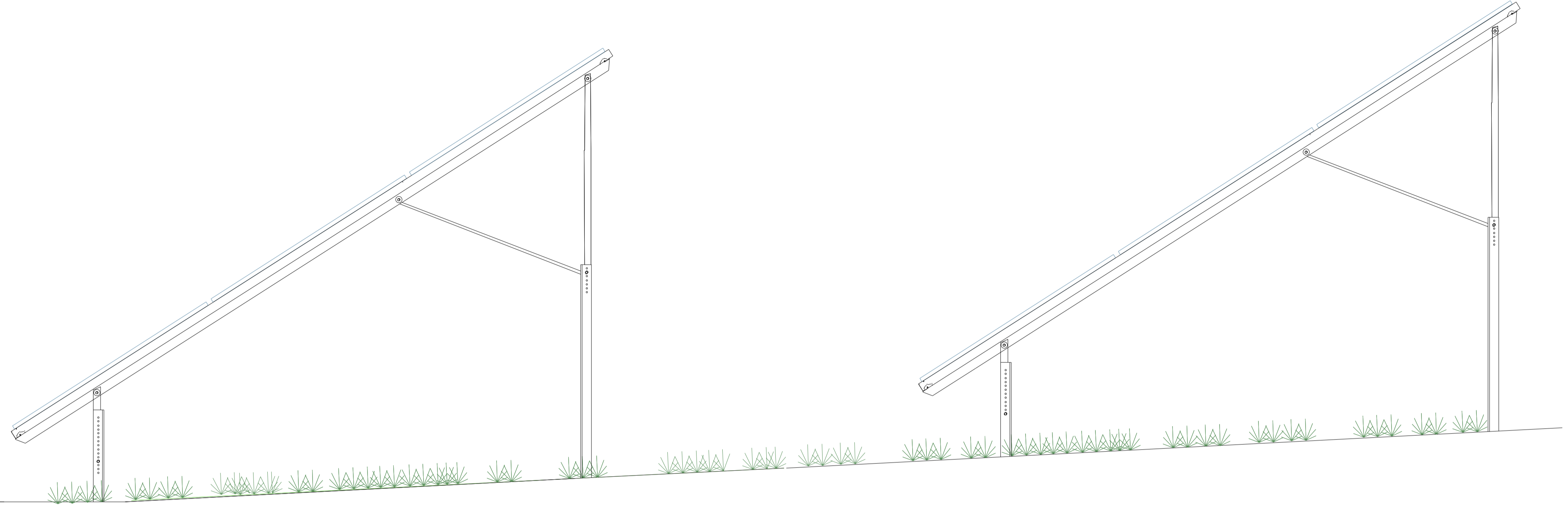
Fasce perimetrali di mitigazione a verde: Sezione tipo longitudinale Scala 1:20
