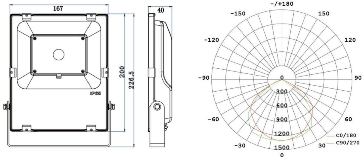
Figura 3.3 - Diagramma fotometrico e viste proiettore
