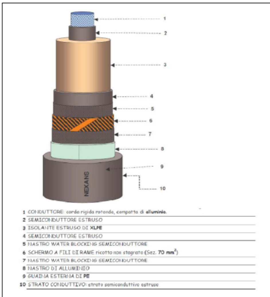
Figura 39 – Schema tipologico del cavo
