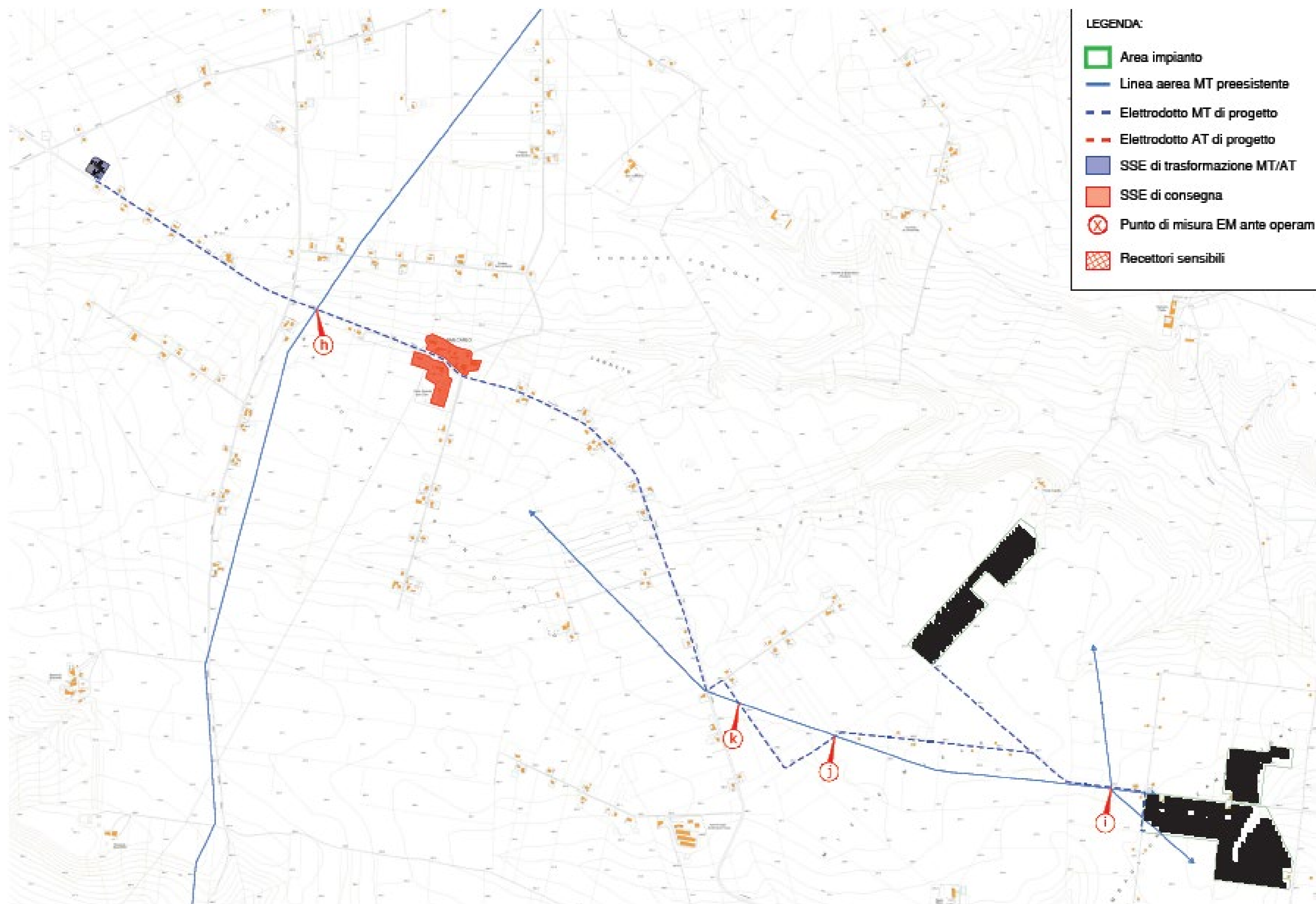
Figura 53 Stralcio planimetrico con rappresentazione del tracciato dell'elettrodotto MT di progetto.
