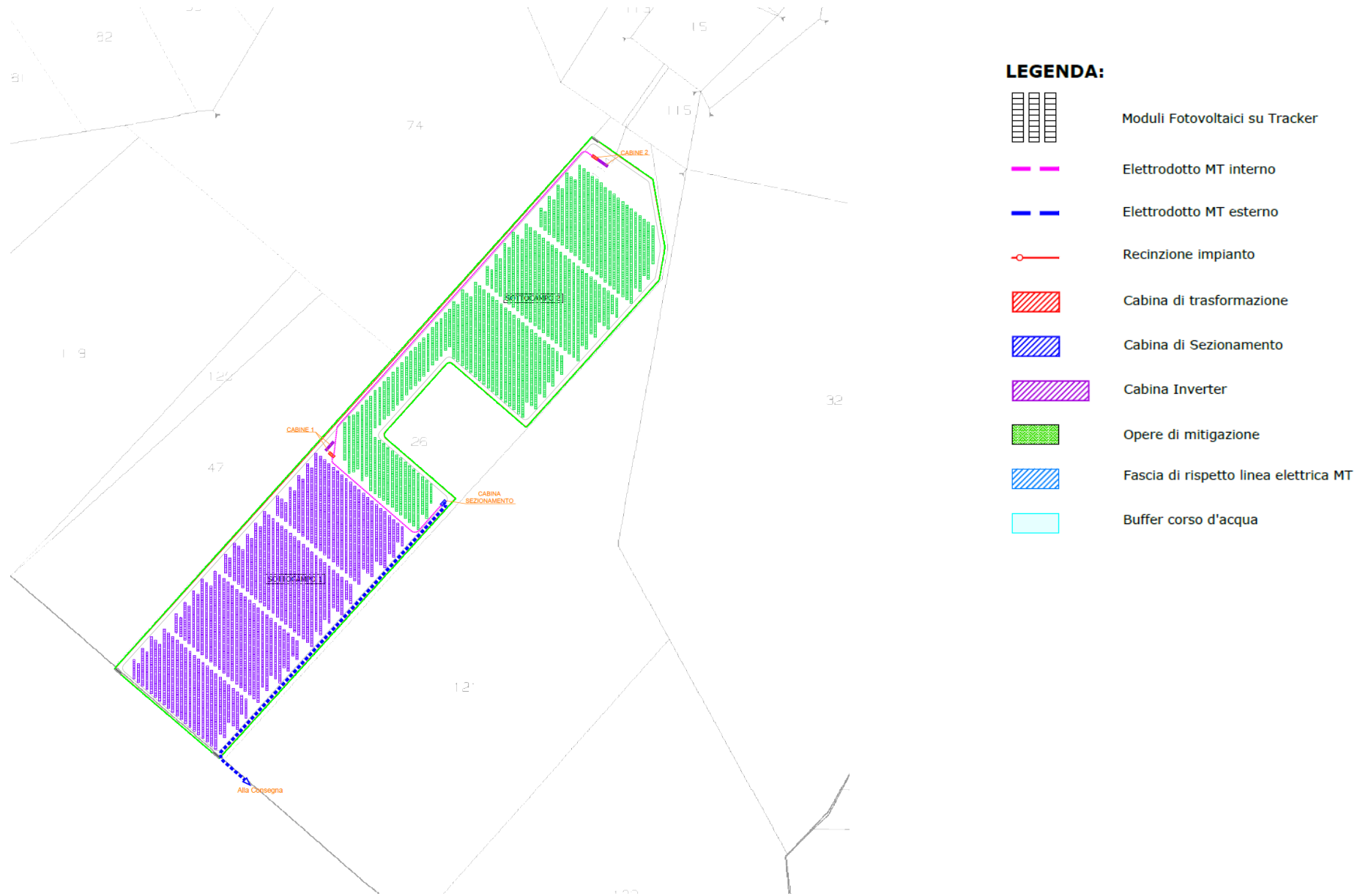
Figura 28a Stralcio elaborato DEF-TAV.07A – Layout impianto con sottocampi
