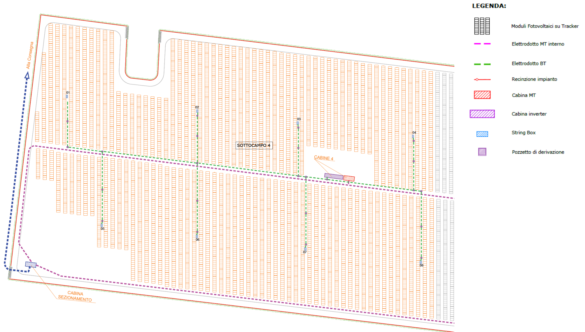
Figura 29 Stralcio elaborato DEF-TAV.12 – Particolare sottocampo
