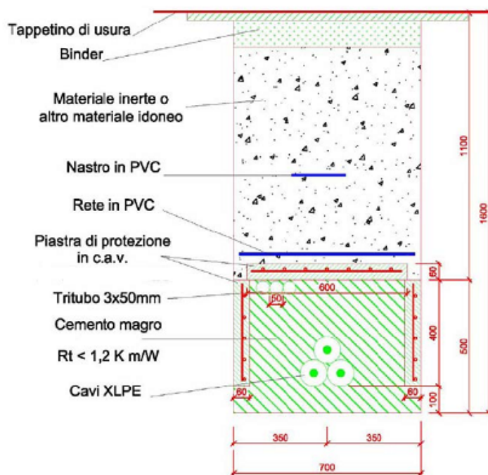
Figura 63 Sezione tipo di posa dei cavi elettrici
