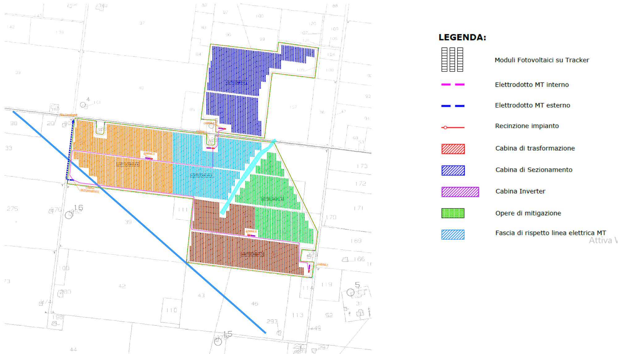
Figura 28b Stralcio elaborato DEF-TAV.07B – Layout impianto con sottocampi
