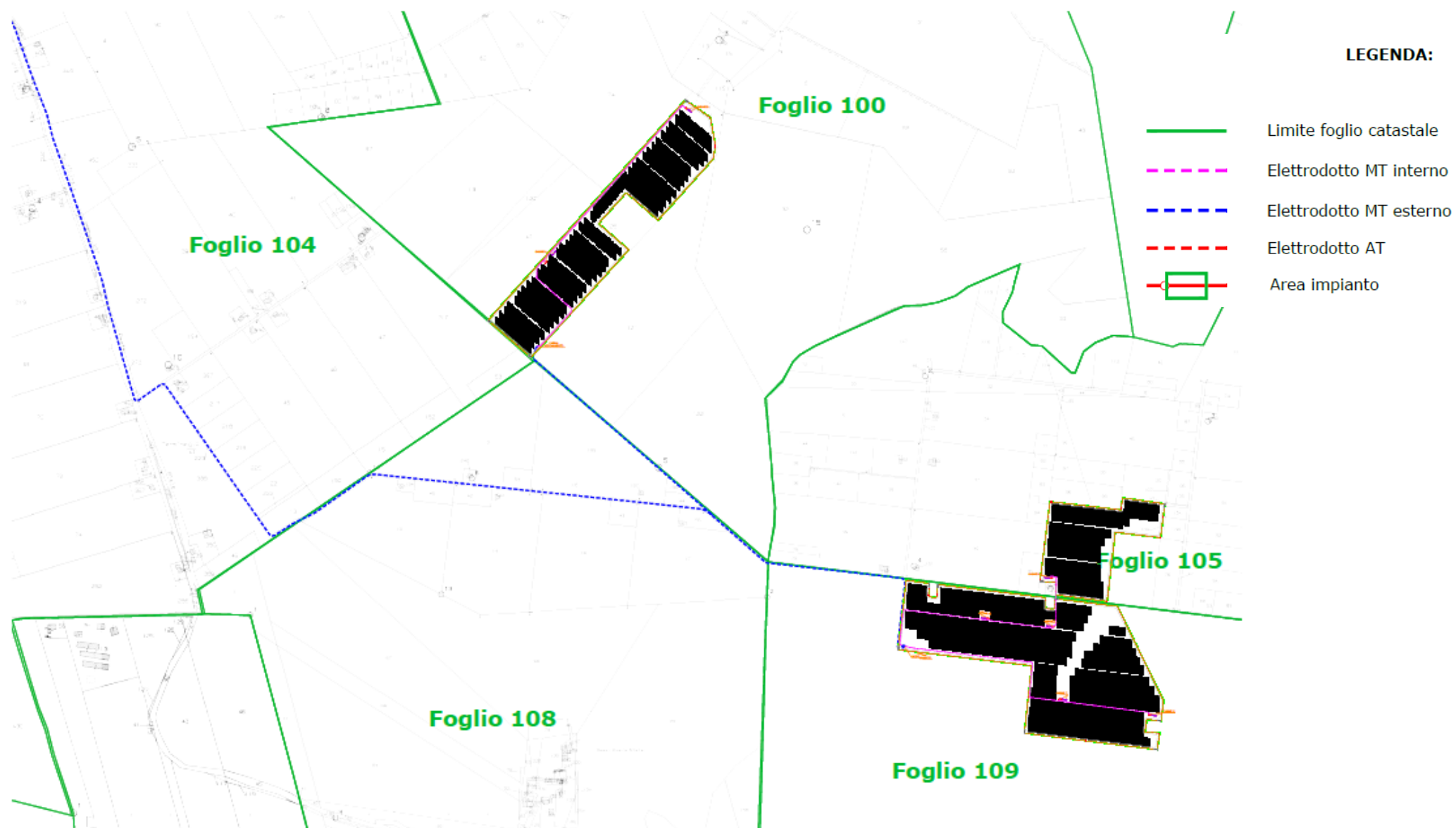
Figura 26 Stralcio elaborato DEF-TAV.06A – Layout su catastale
