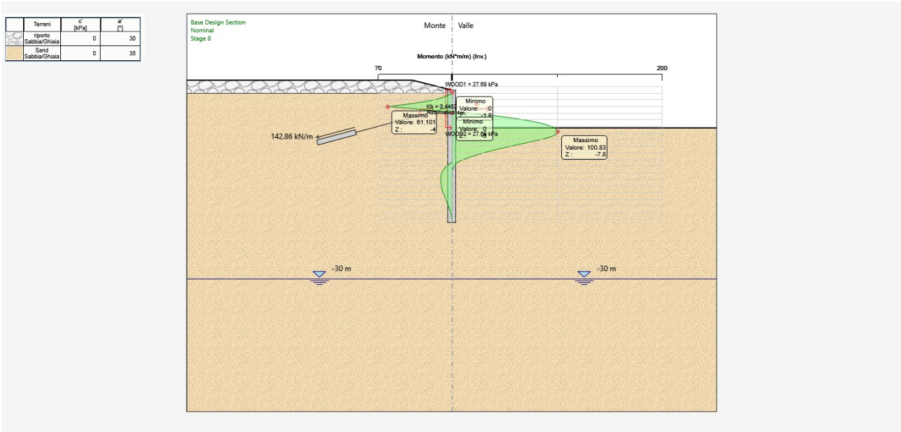
Involuppo fasi statiche - SLE – momenti flettenti.
