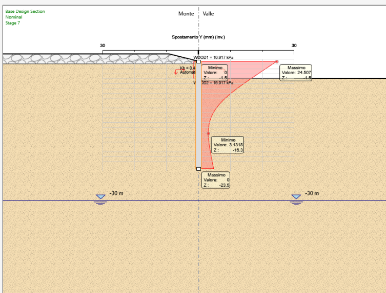
Combinazione sismica – deformata.
