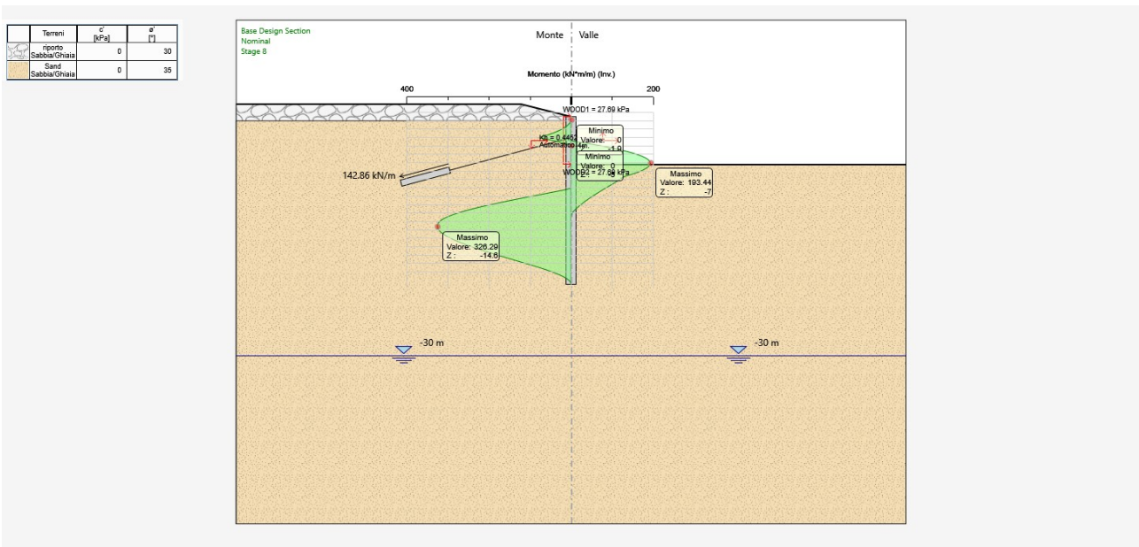
Combinazione sismica – momenti flettenti.
