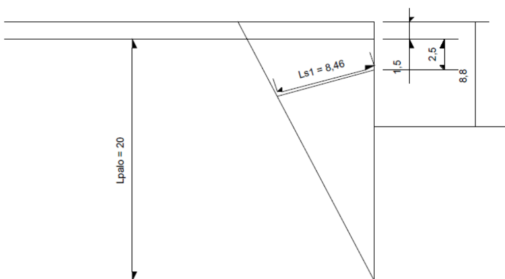
Figura 2: metodo grafico per il calcolo della lunghezza libera di ancoraggio
