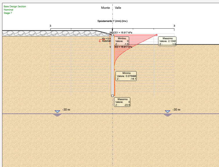
Involuppo fasi statiche - SLE- deformata.
