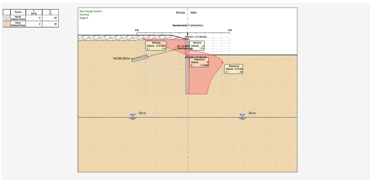
Inviluppo fasi statiche - SLE- deformata.
