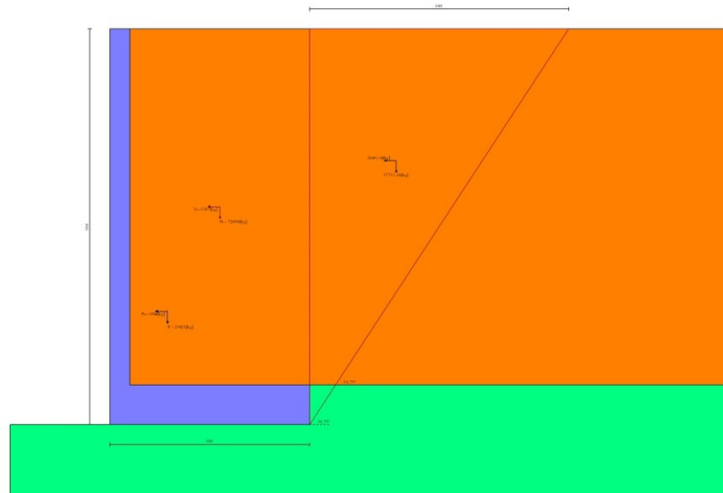
Fig. 5 - Cuneo di spinta (combinazione sismica) (Combinazione n° 1)
