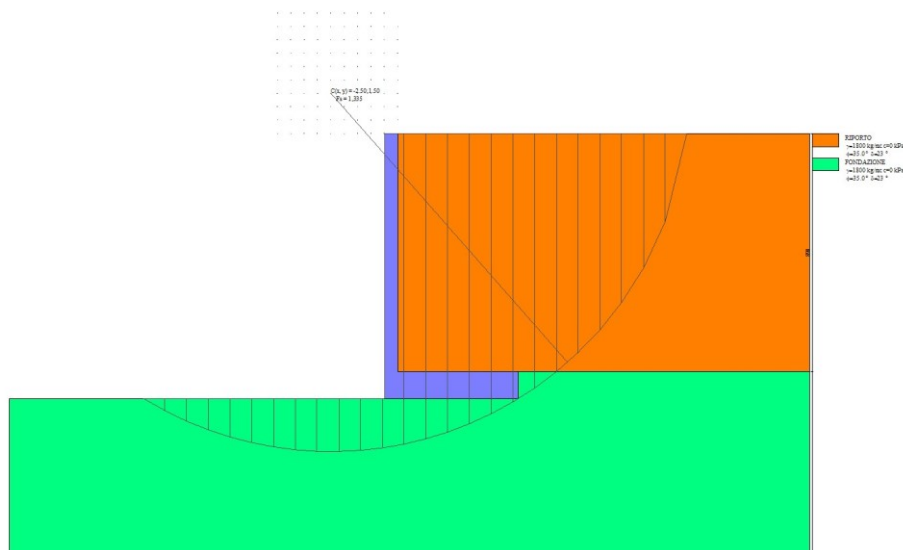
Fig. 12 - Stabilità fronte di scavo - Cerchio critico (Combinazione n° 8)
