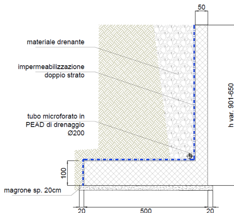
Figura 2: Sezione trasversale muro di sostegno
