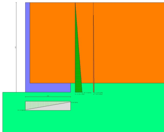
Fig. 6 - Diagramma delle pressioni (combinazione sismica) (Combinazione n° 1)
