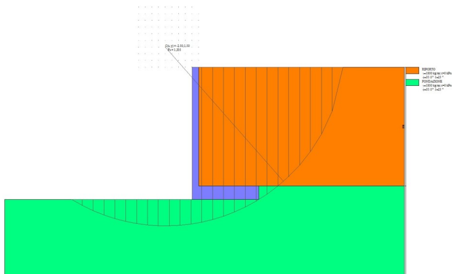
Fig. 7 - Stabilità fronte di scavo - Cerchio critico (Combinazione n° 8)
